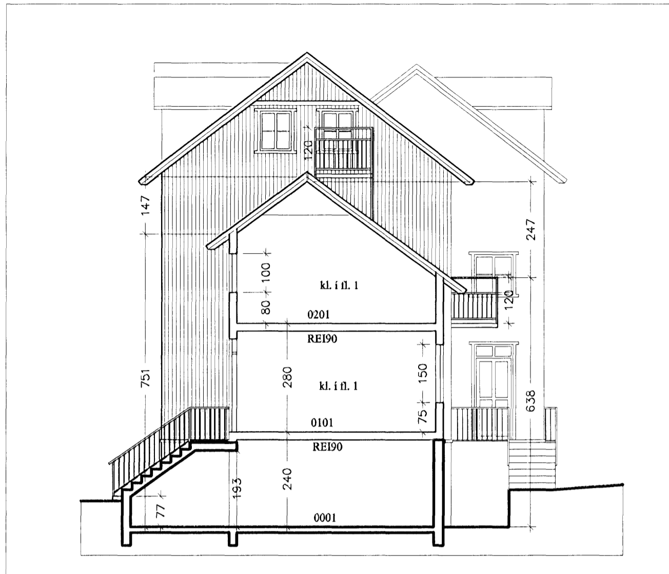
Sneiðing b-b 1:100
