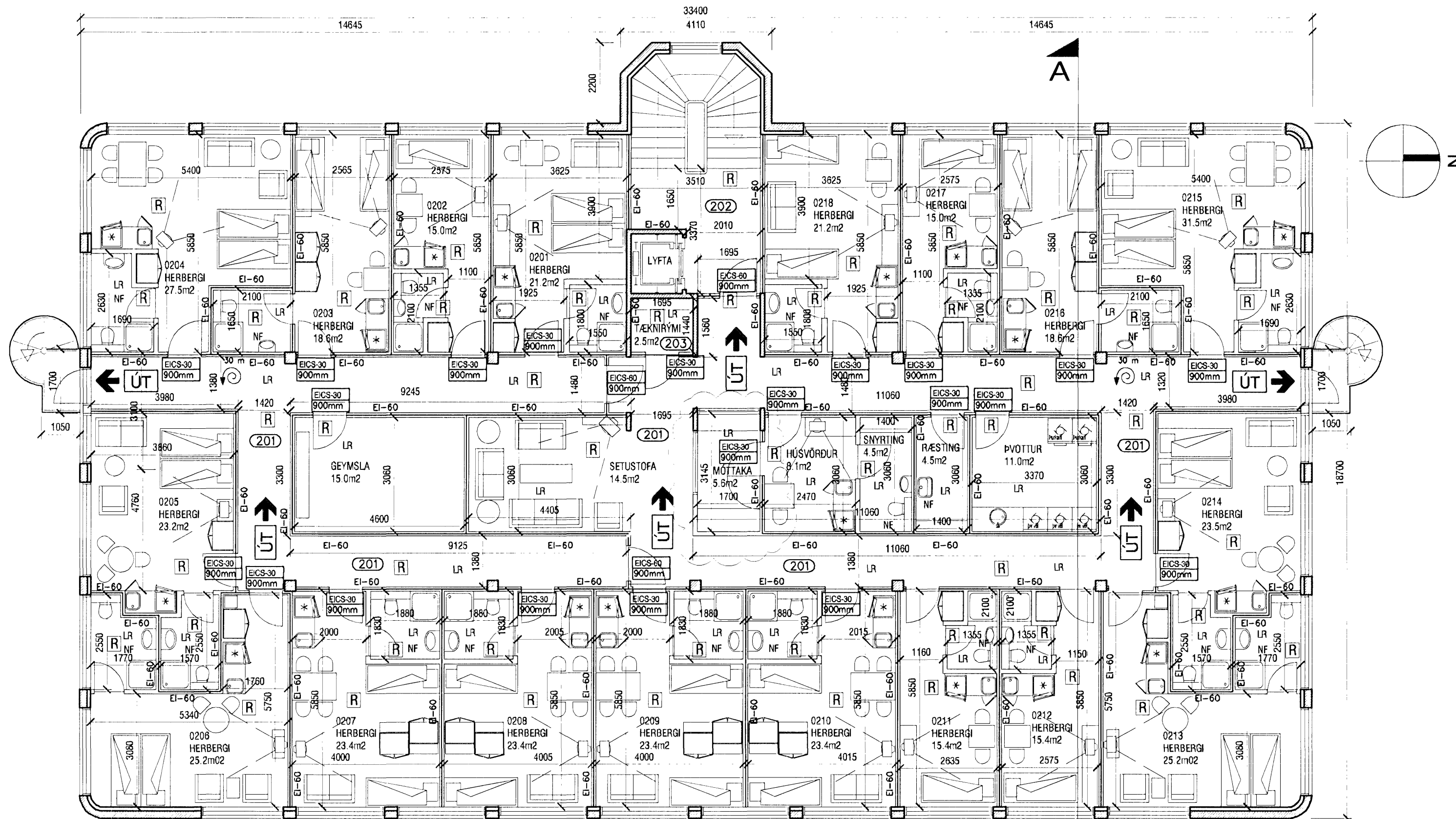
A Grunnmynd 2. hæðar mkv. 1:100
