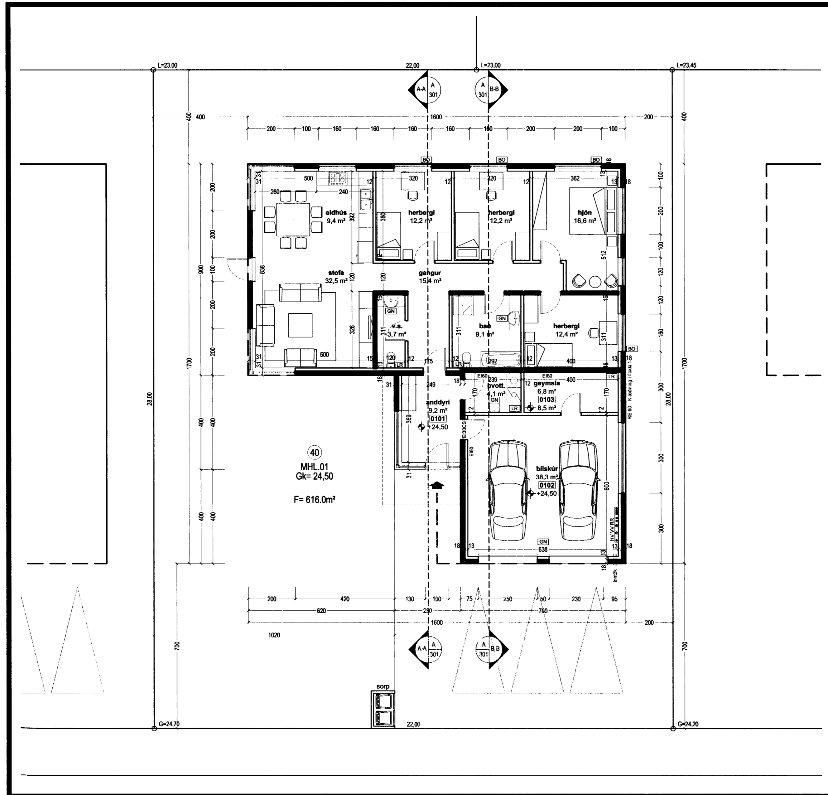
Grunnmynd 1:100
