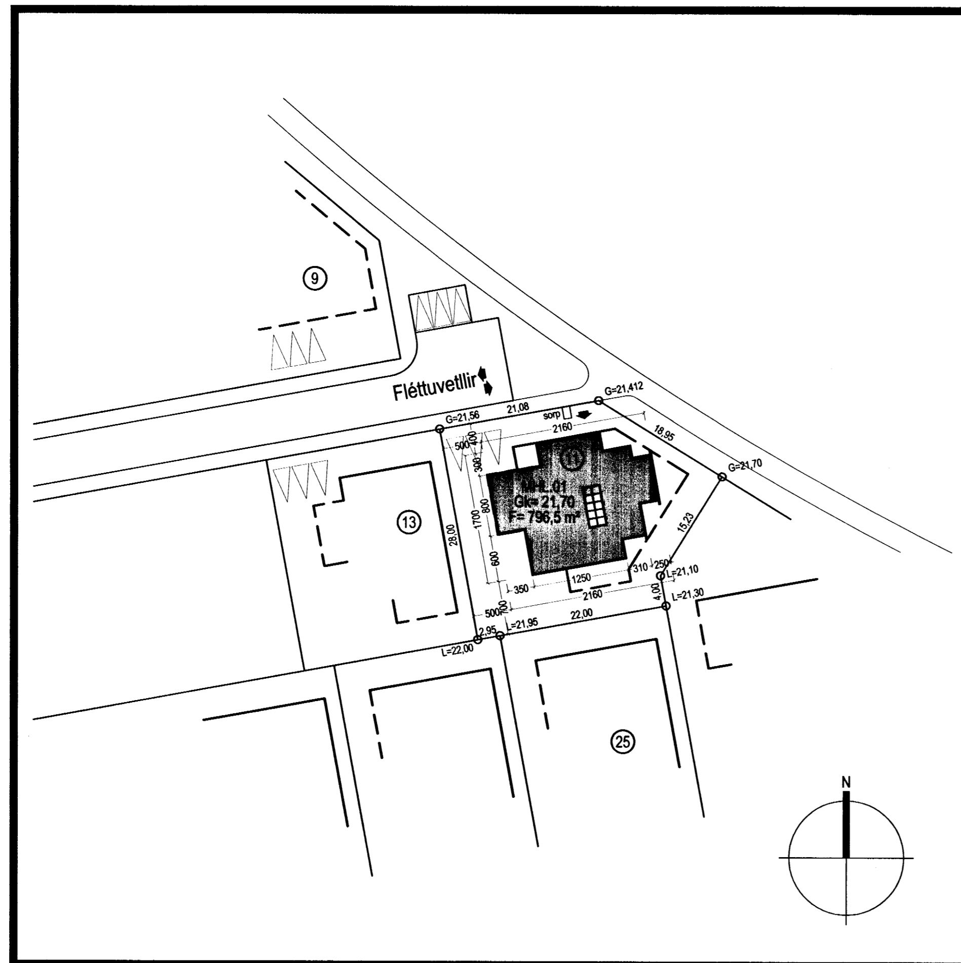
Afstöðumynd 1:500
