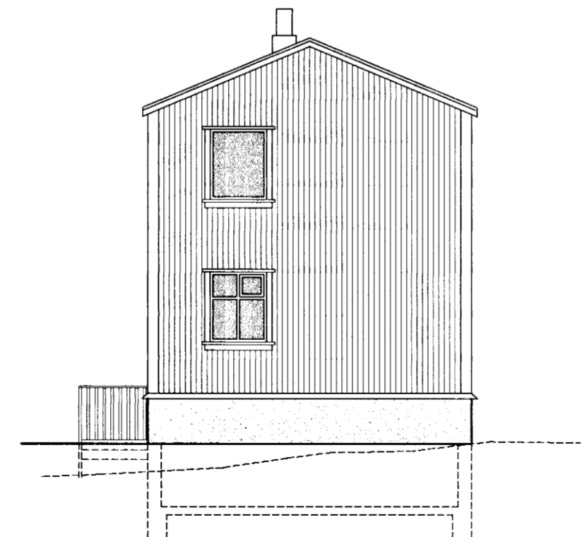
ÚTLIT VESTUR
