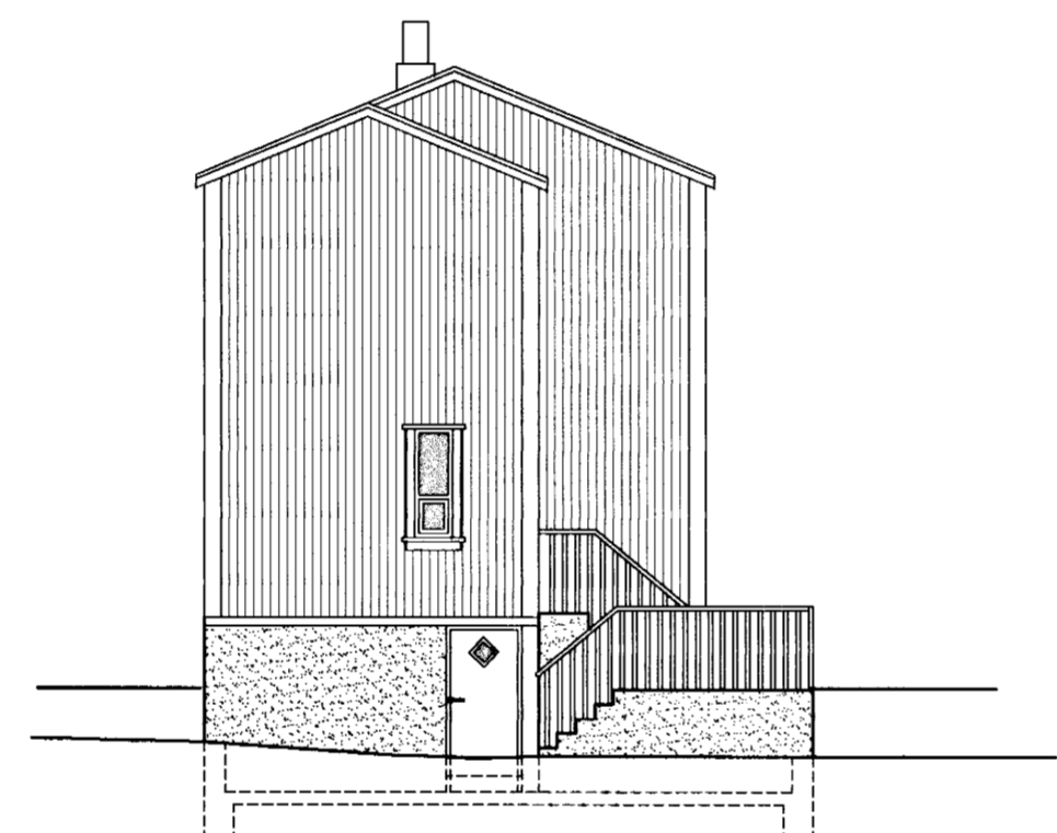
ÚTLIT AUSTUR
