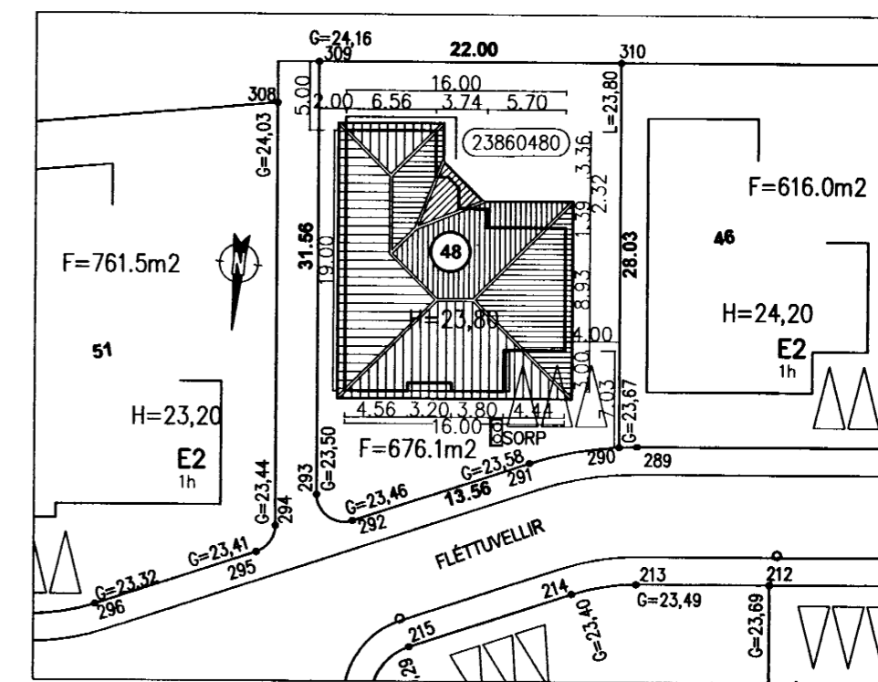
AFSTÖÐUMYND 1:500
