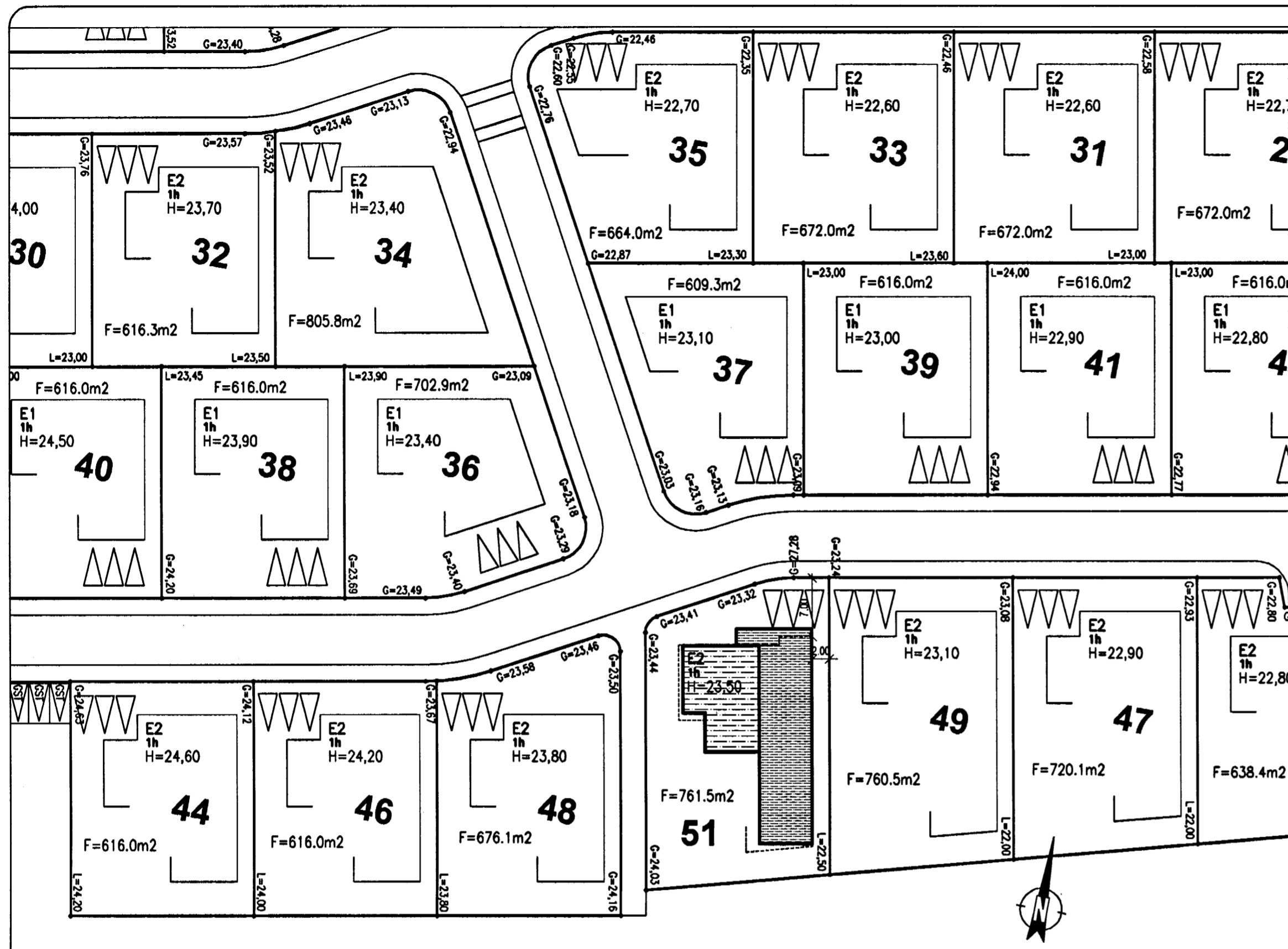
AFSTÖÐUMYND 1:500
