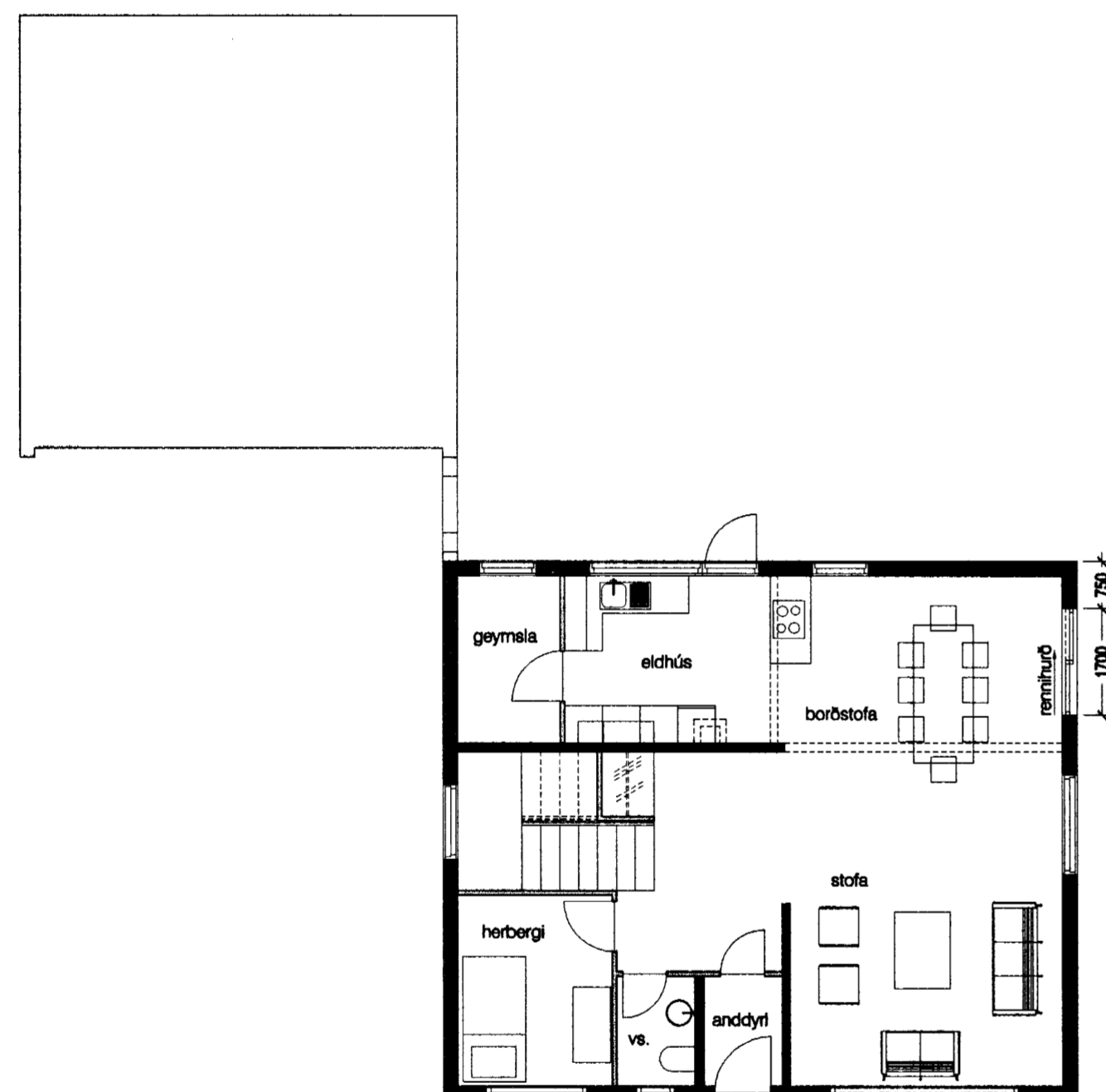
grunnmynd 1.hæðar
