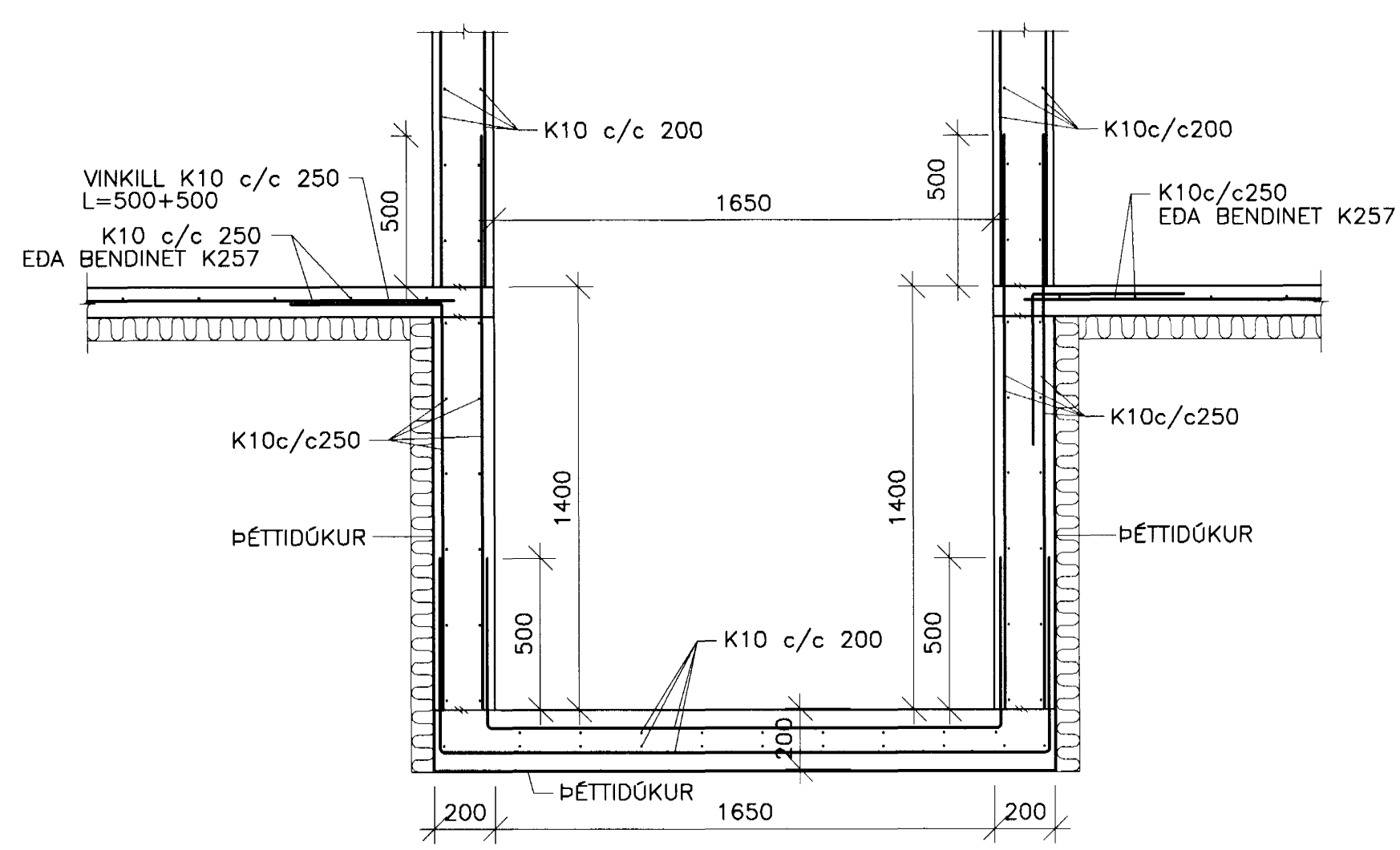
30 SNID 201 1:20
