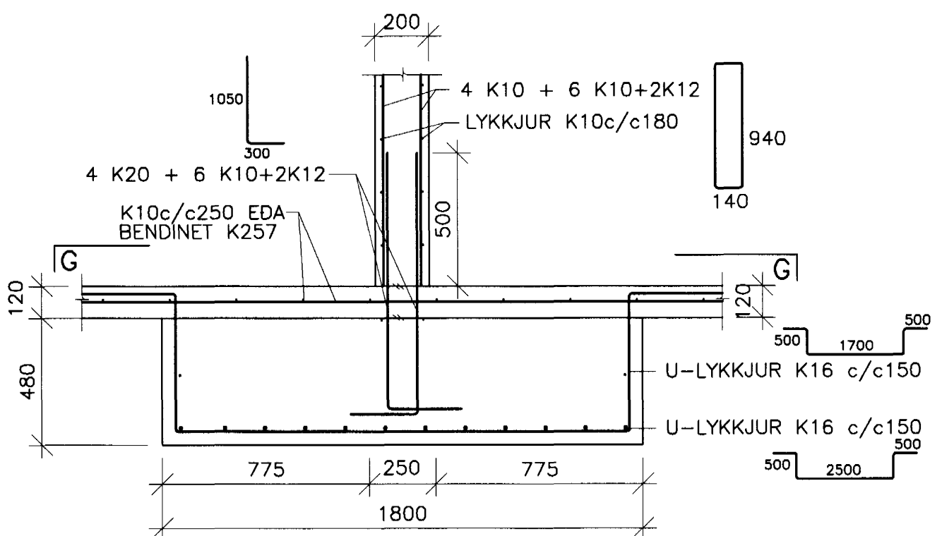
26 SNID 201 1:20
