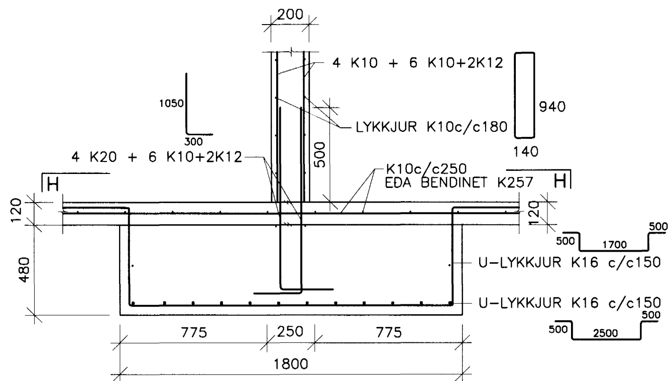
27 SNID 201 1:20
