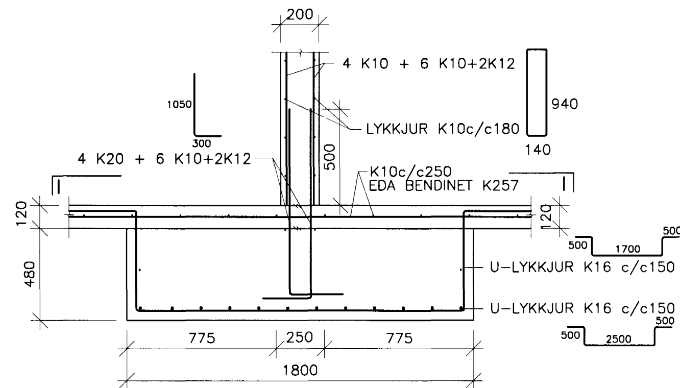
28 SNID 201 1:20
