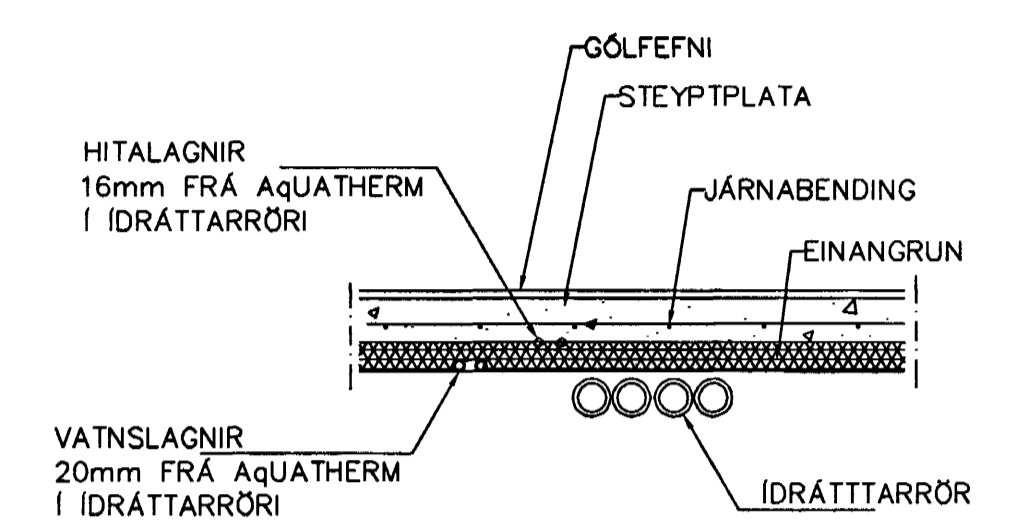
LAGNIR, SNIÐ, 1:20
