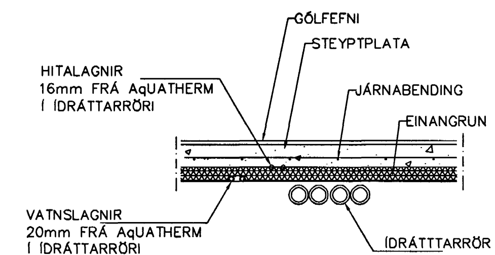
LAGNIR, SNIÐ, 1:20
