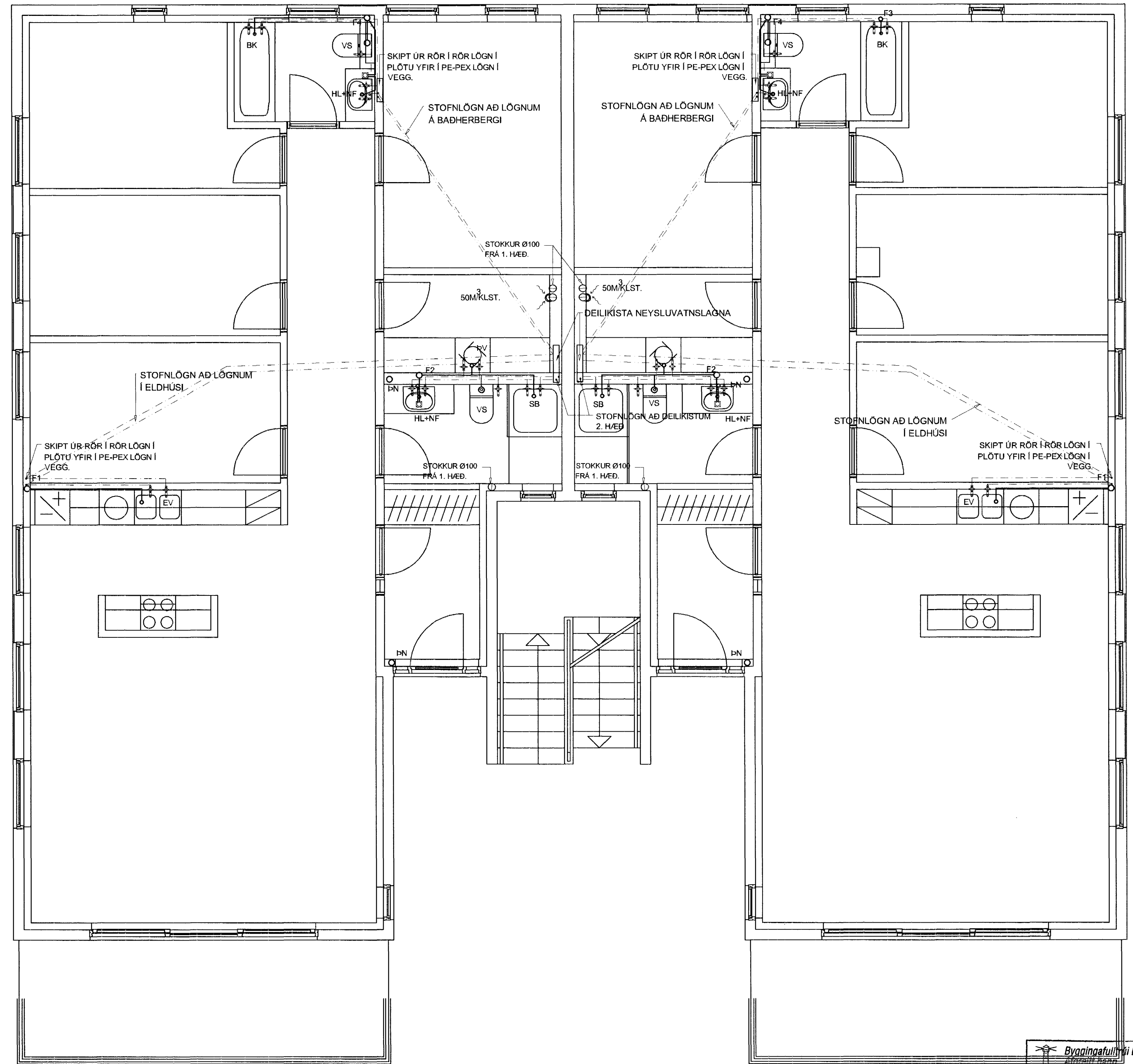
GRUNNMYND NEYSLUVATNSLAGNA 2. HÆÐ, 1:50 GRUNNMYND LOFTRÆSILAGNA 2. HÆÐ, 1:50
