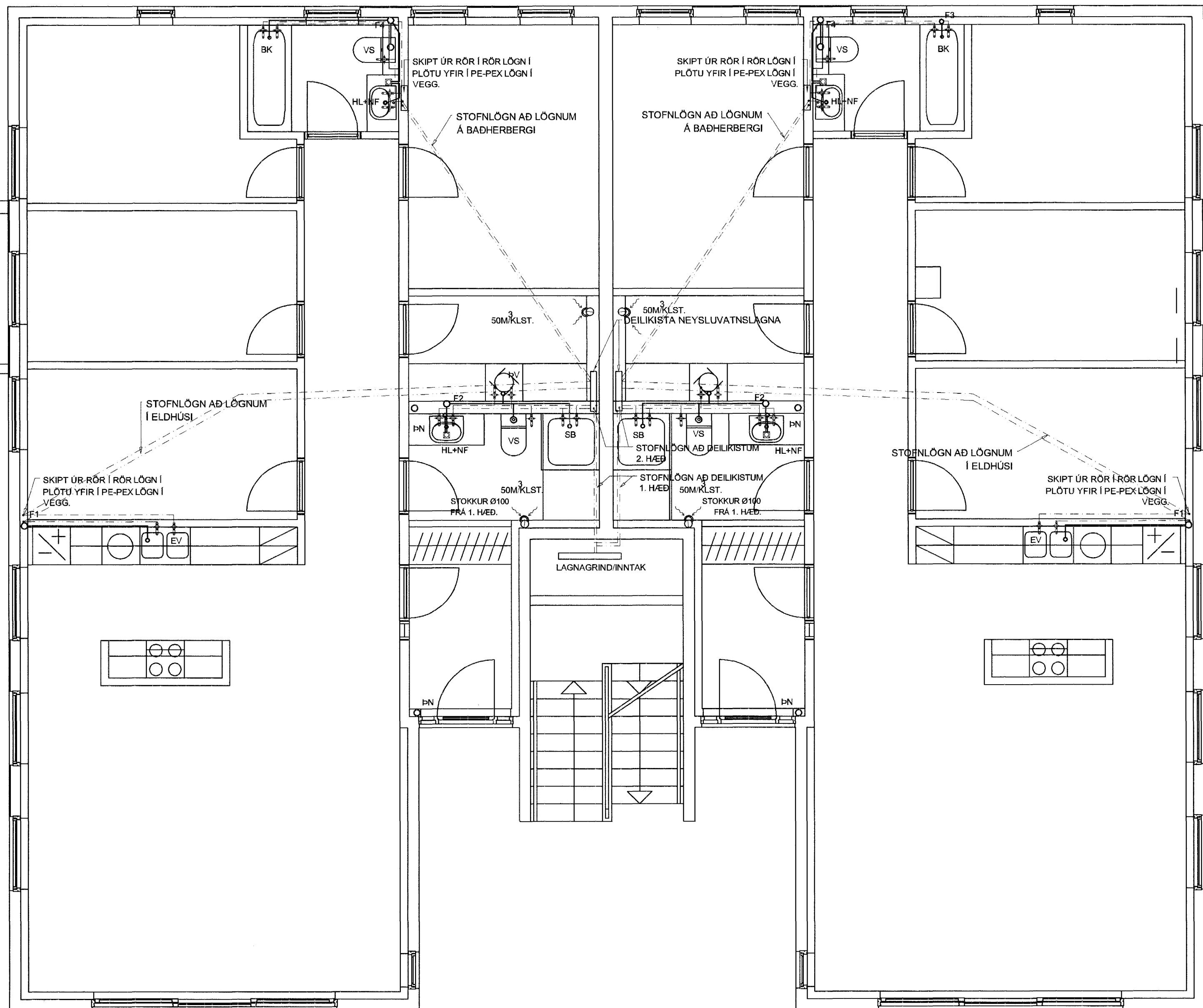
GRUNNMYND NEYSLUVATNSLAGNA 1. HÆÐ, 1:50 GRUNNMYND LOFTRÆSILAGNA 1. HÆÐ, 1:50
