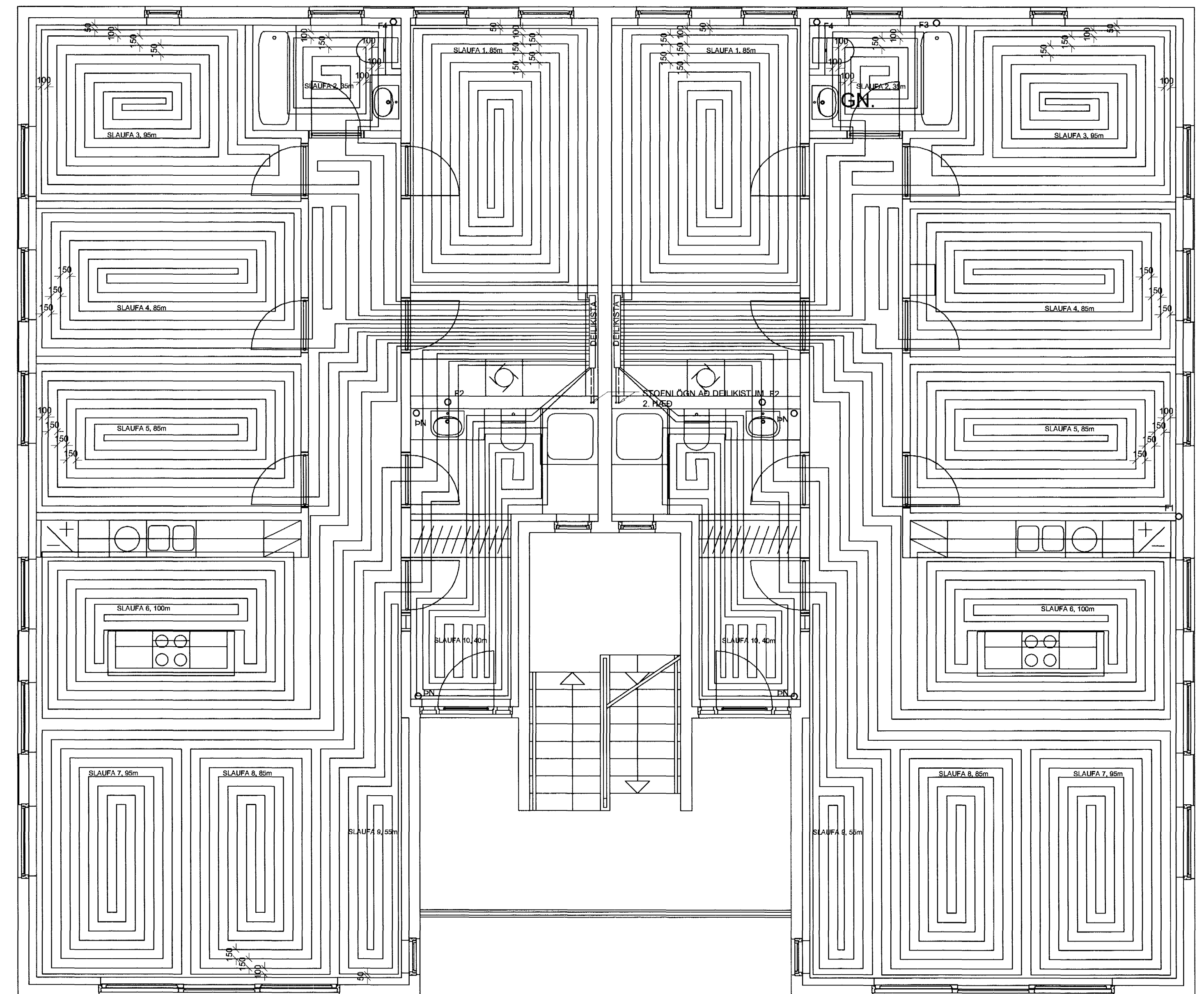
GRUNNMYND GÓLFHITALAGNA 2. HÆÐ, 1:50
