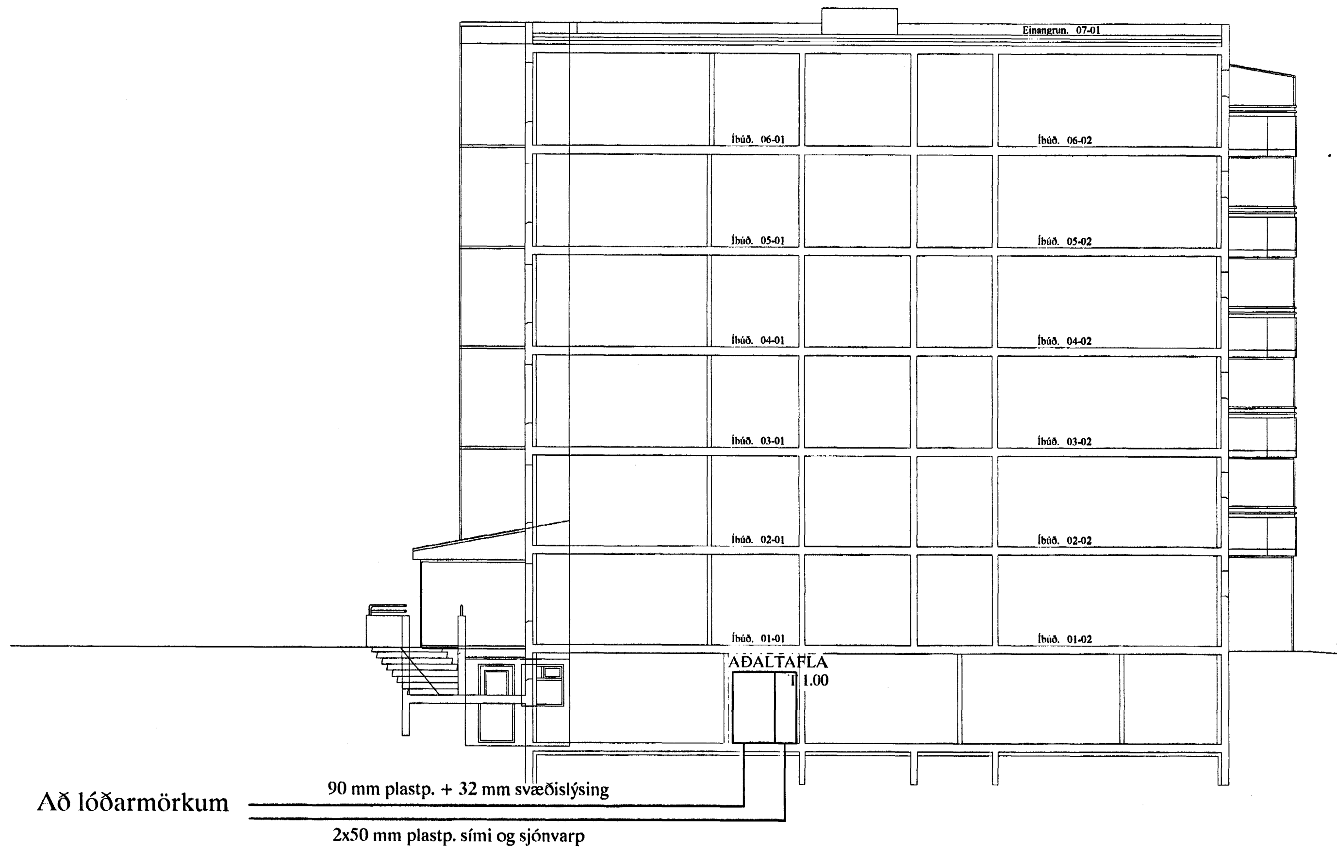
SNIÐ Í INNTAK M. 1:100
