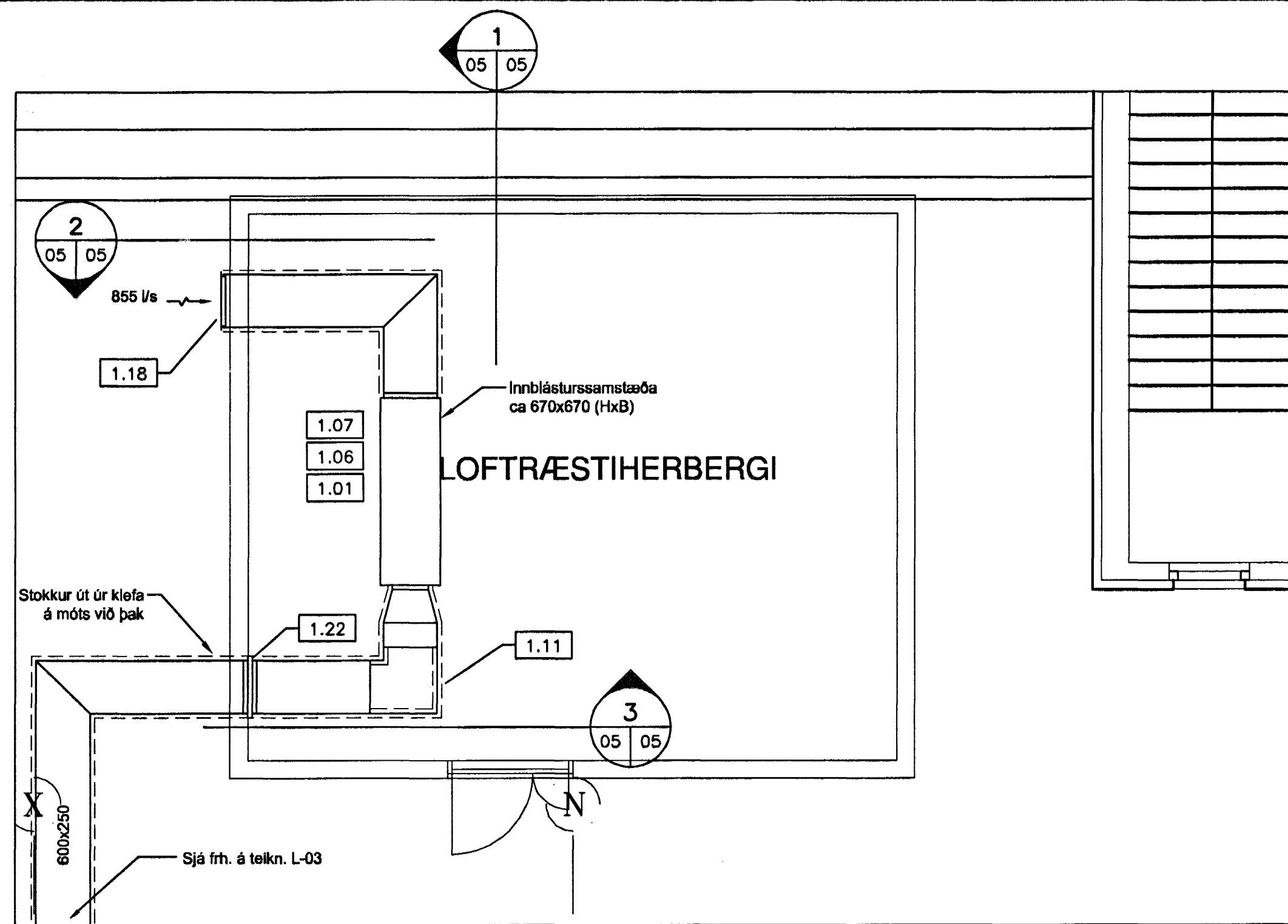
GRUNNMYND – LOFTRÆSIKLEFI M. 1:50
