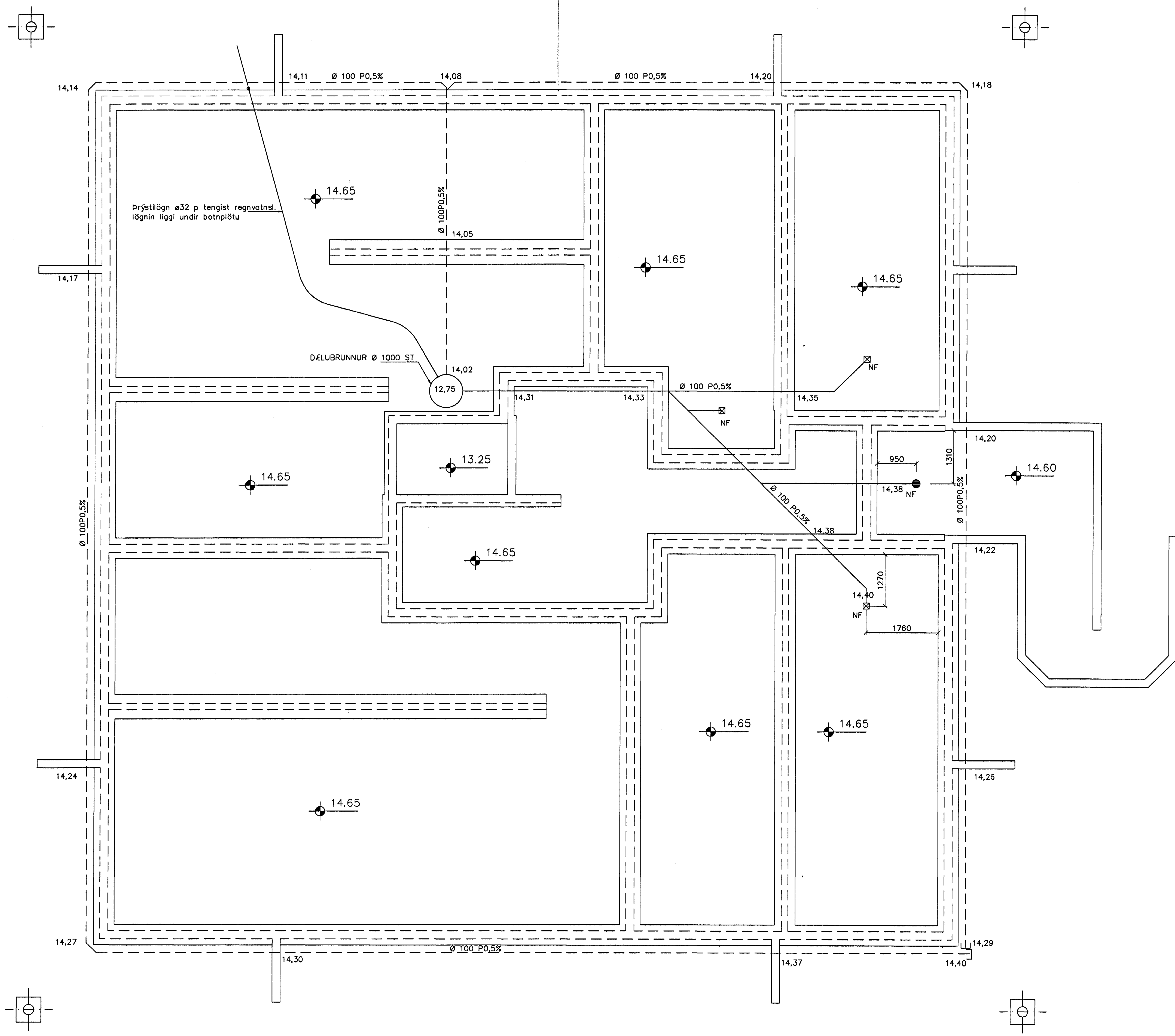
GRUNNMYND 1:50
