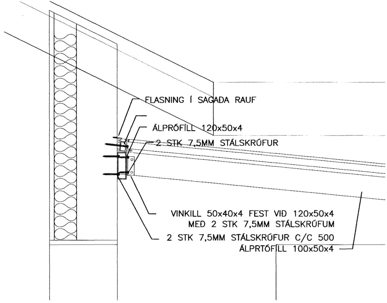
DEILL D 1:10
