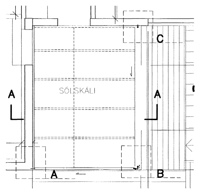
GRUNNMYND. SÓLSKÁLI 1:50
