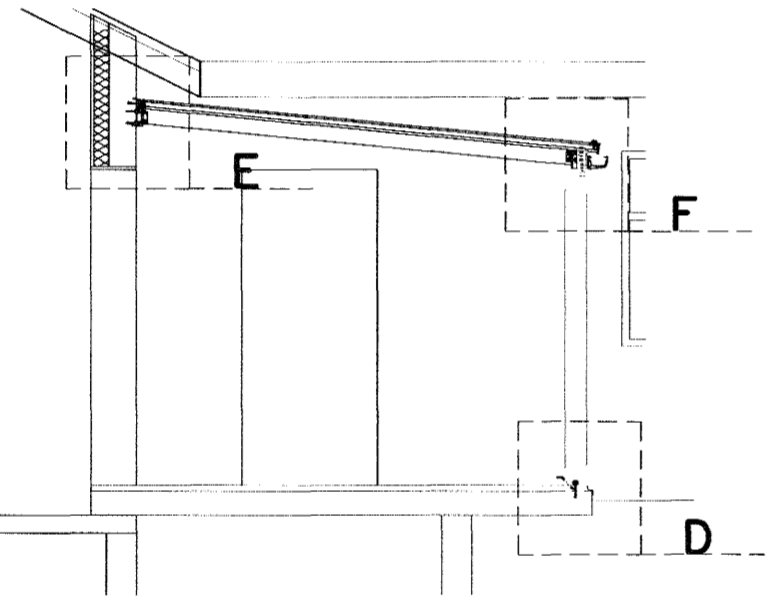
SNID A-A 1:50
