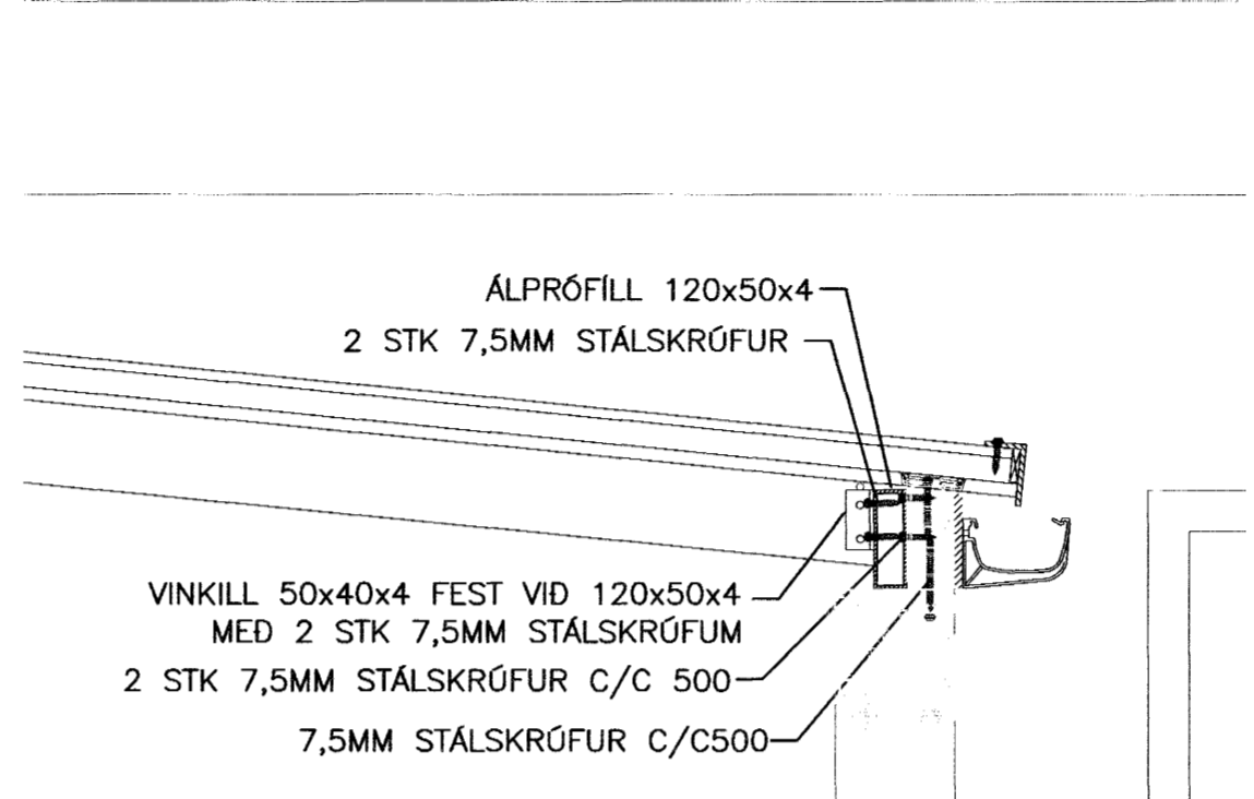
DEILL E 1:10
