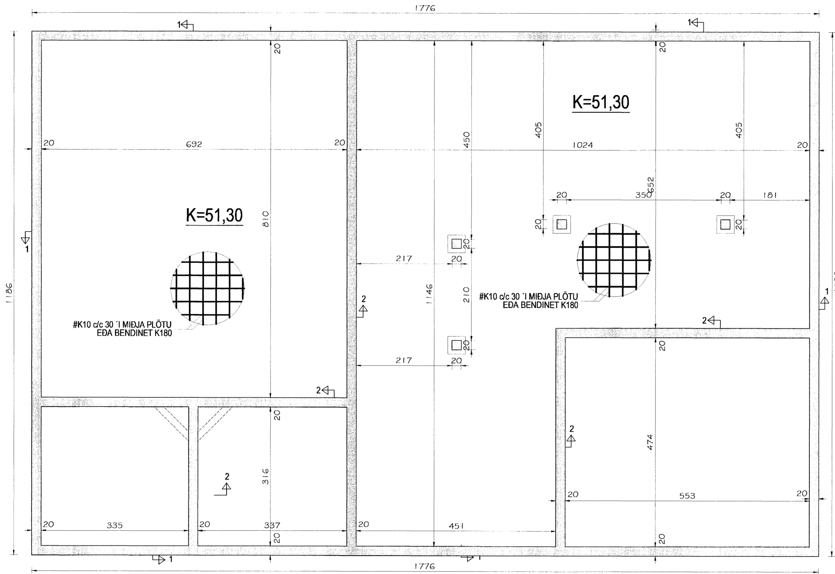
GRUNNMYND SÖKKLA MKV. 1:50
