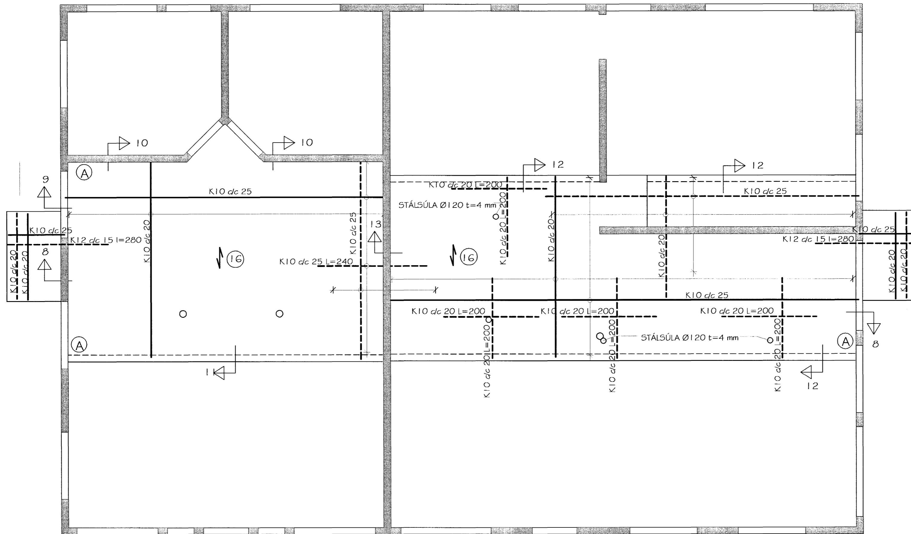
JÁRN Í GÓLFPLÖTU EFRI HÆÐAR GRUNNMYND MKV. 1:50
