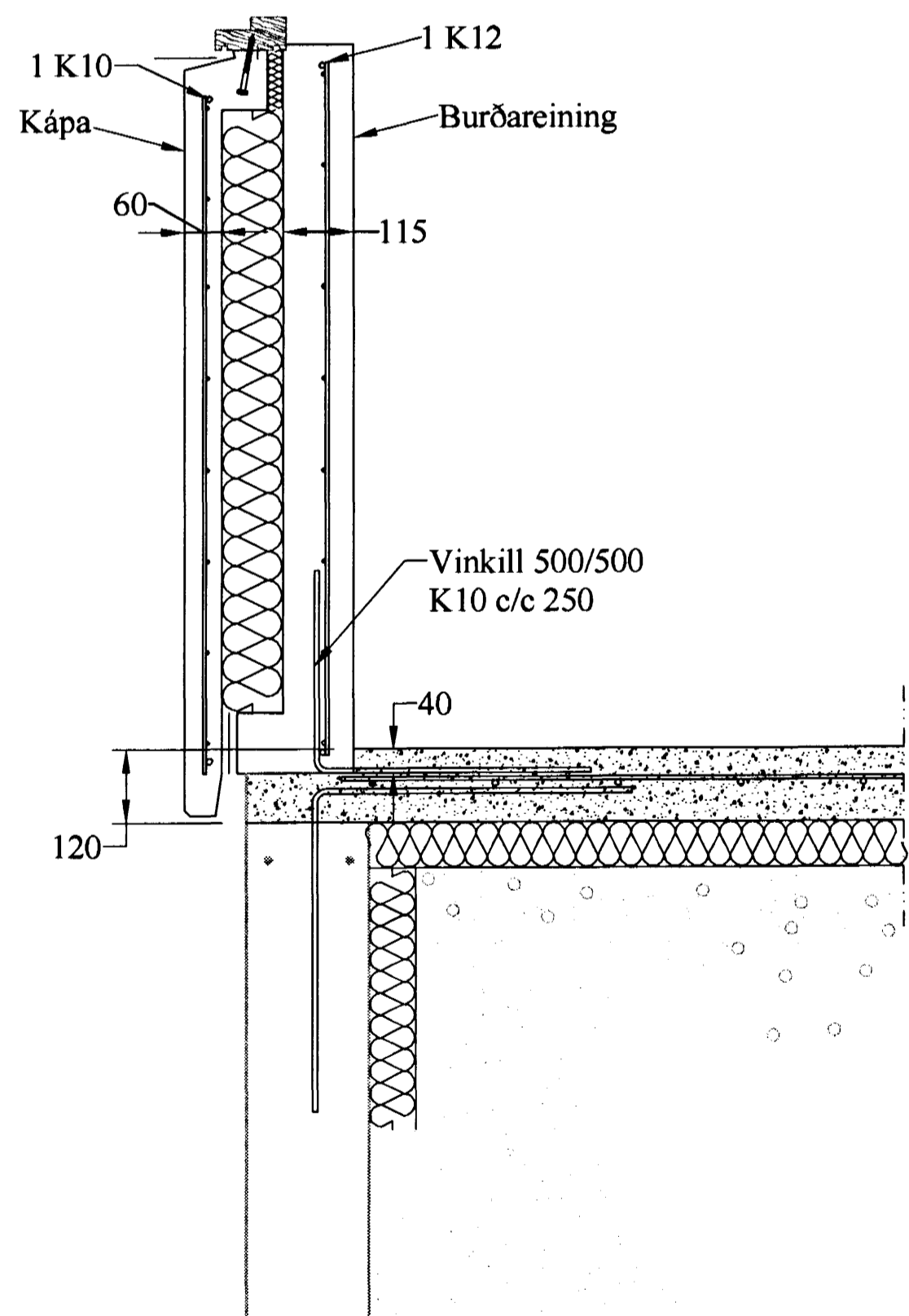
Snið 1 1:20 1-03
