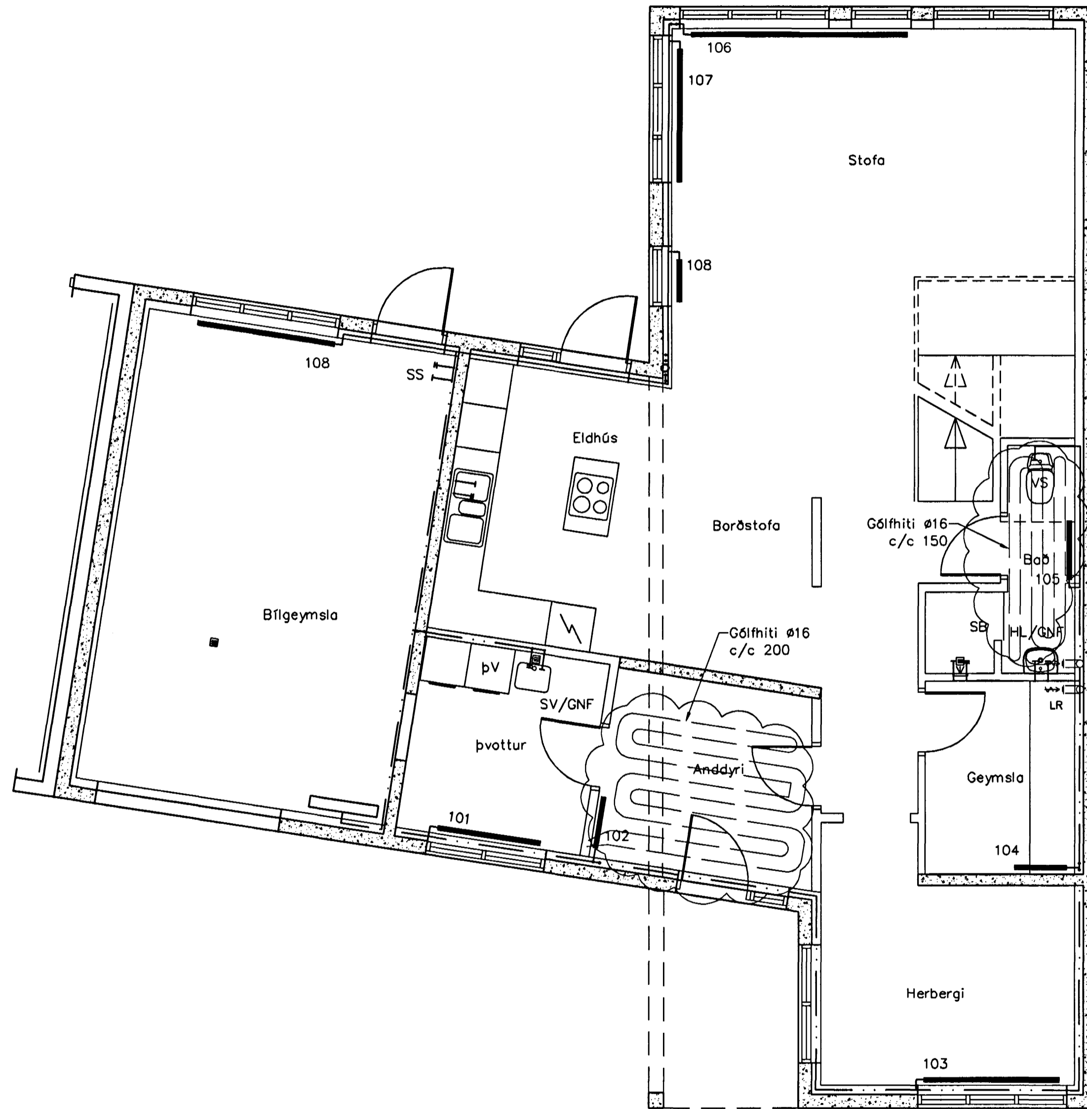
Lagnir 1. hæð, 1:50
