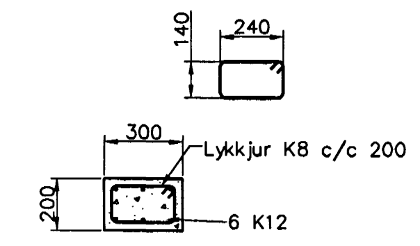
Sála S.1 1:20 1-03
