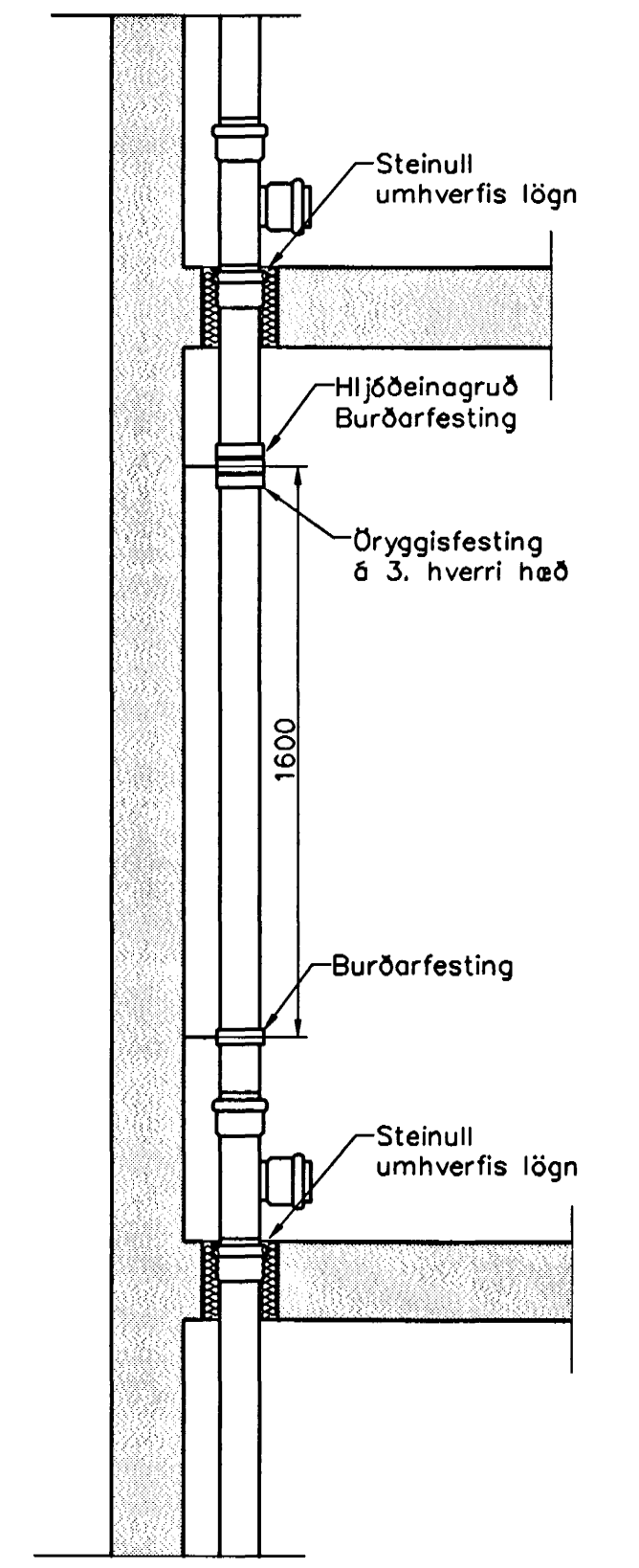
Fallpípa, festingar 1:20
