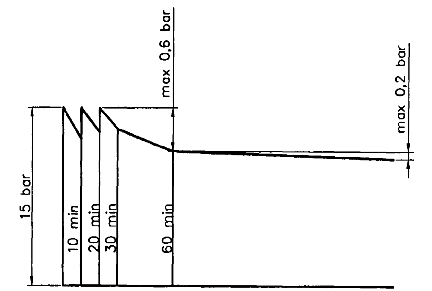
Þrjúþípröfun á neysluvatnslögnum línurit
