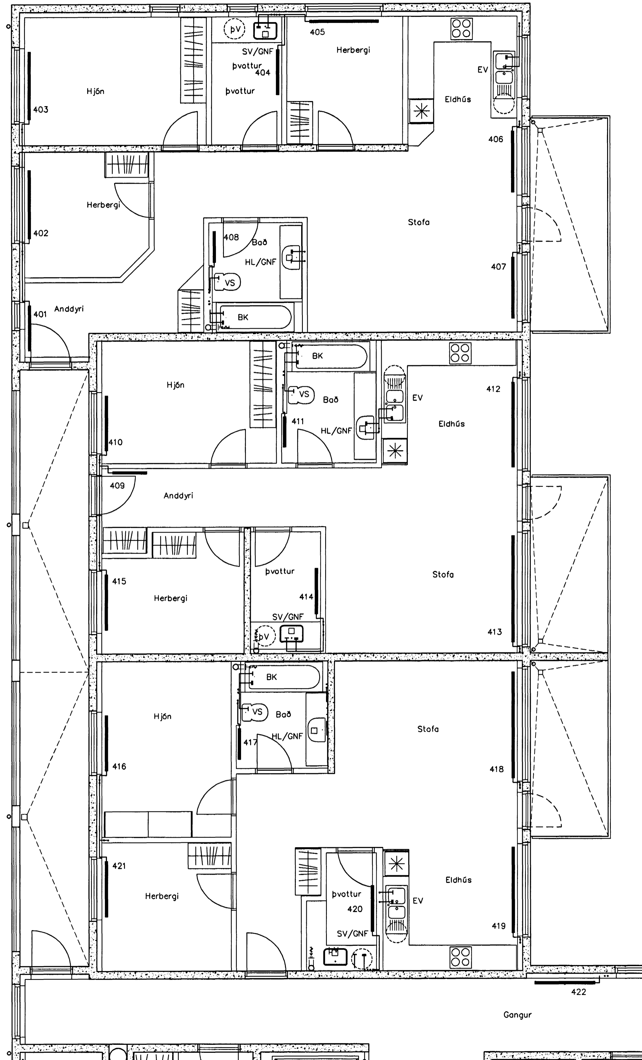
Lagnir 4. hæð, Grunnmynd, 1:50
