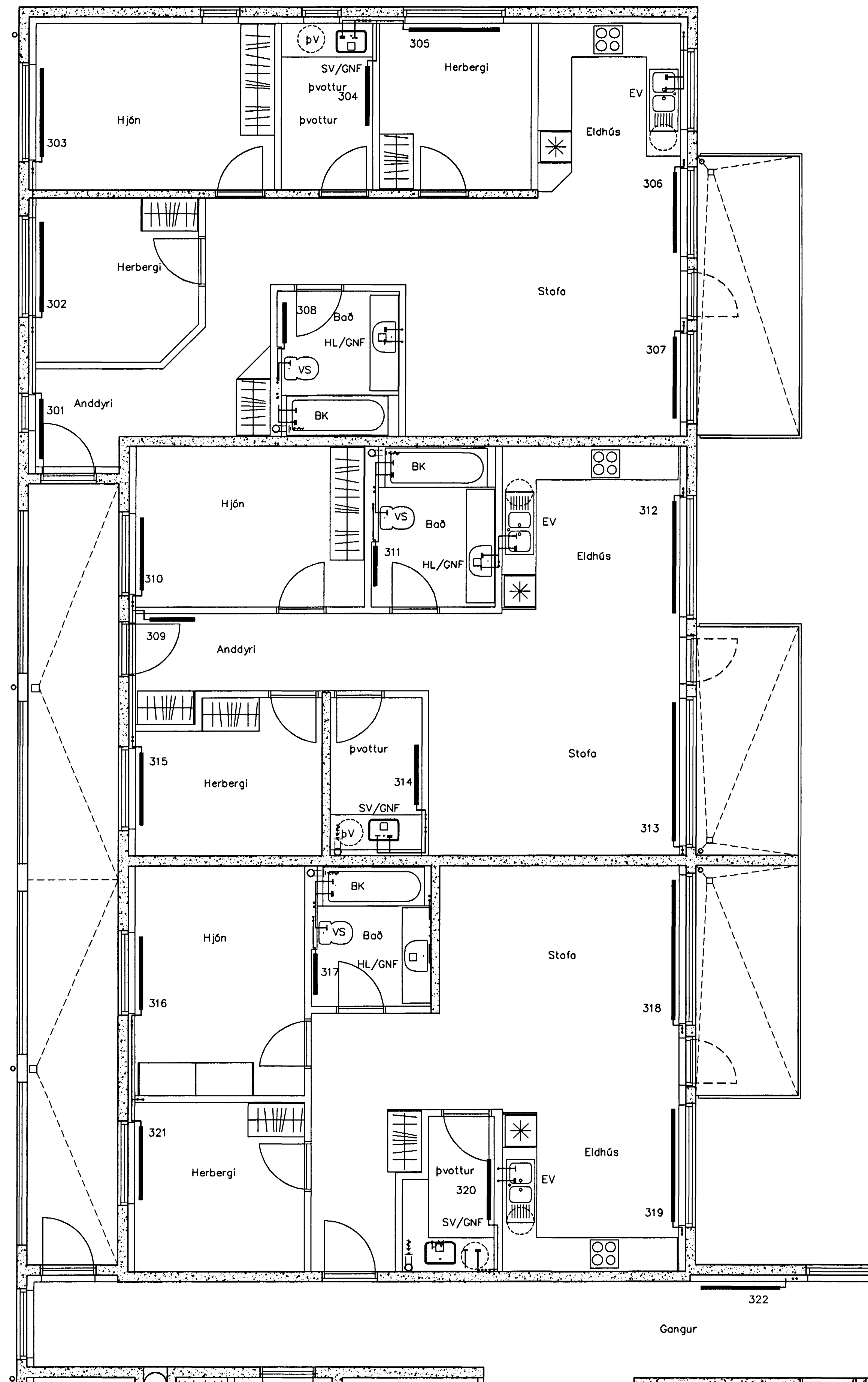
Lagnir 3. hæð, Grunnmynd, 1:50
