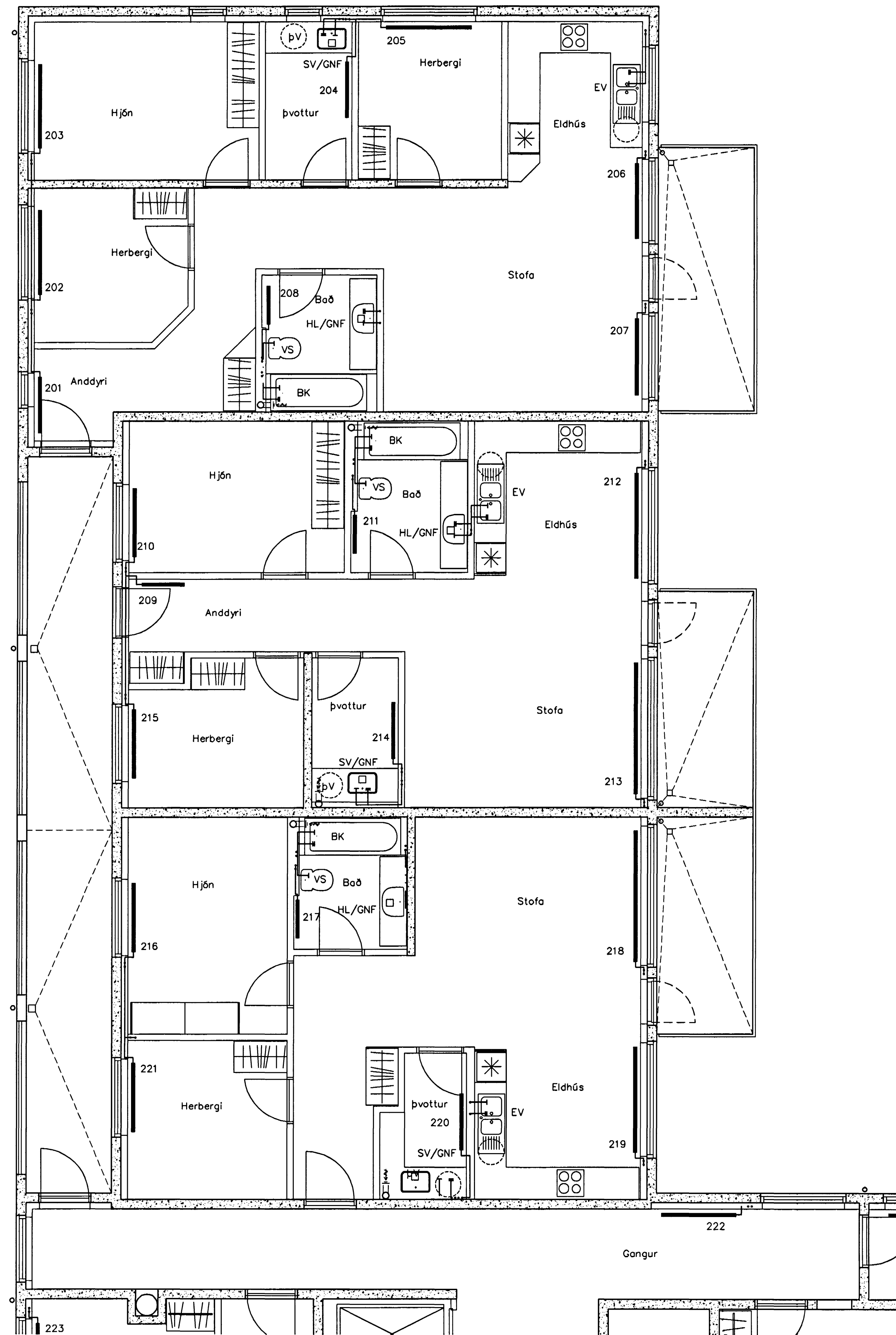
Lagnir 2. hæð, Grunnmynd, 1:50
