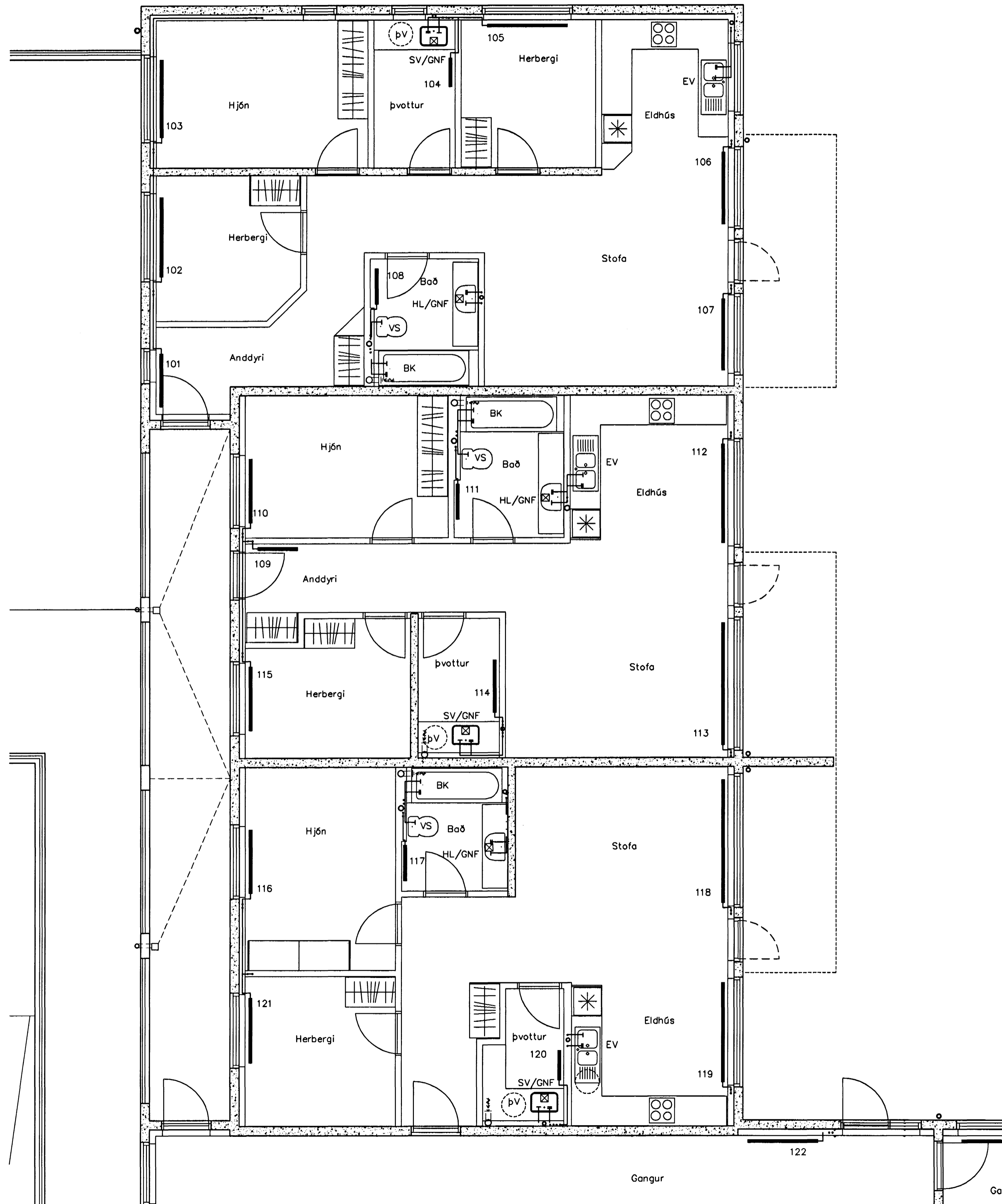
Lagnir 1. hæð, Grunnmynd, 1:50
