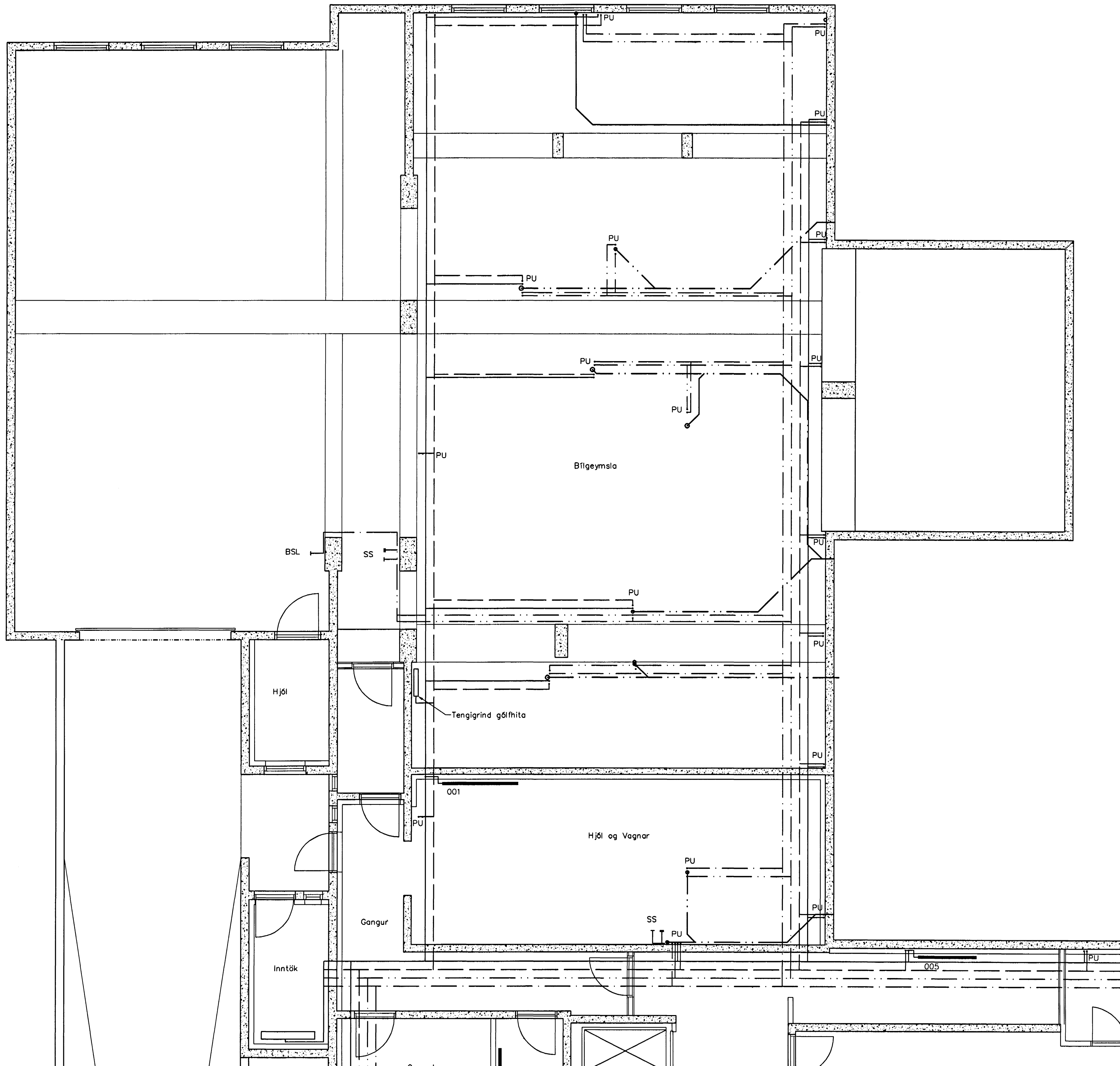
Lagnir kjallara, Grunnmynd, 1:50
