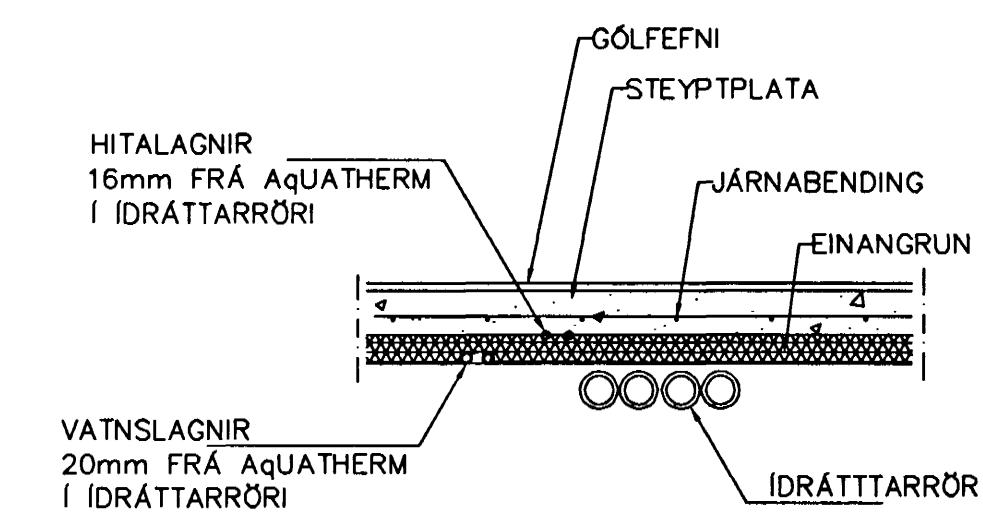
LAGNIR, SNIÐ, 1:20
