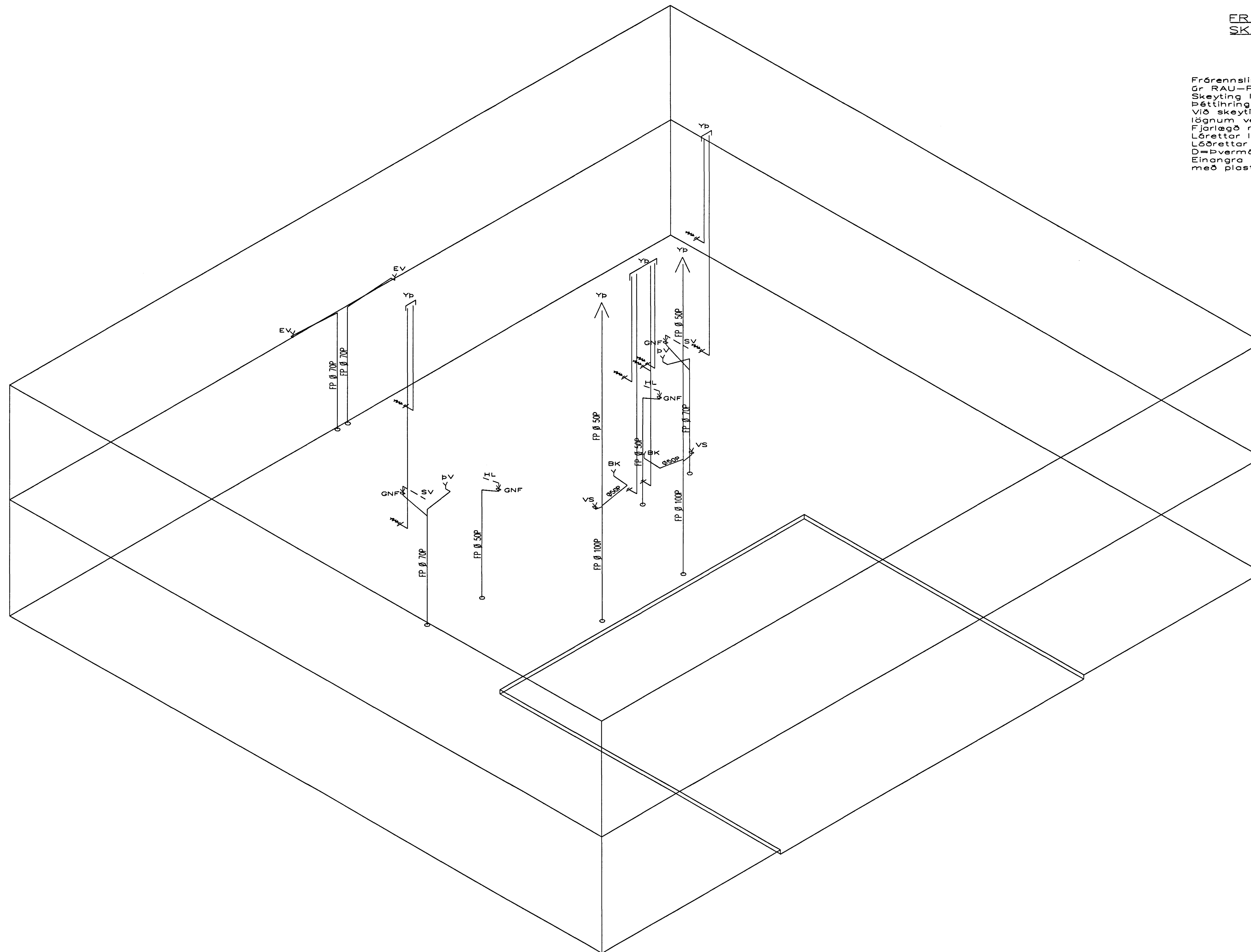
RÚMMYND FRÆRENNSLIS OG LOFTRÆSTILAGNA 1:50
