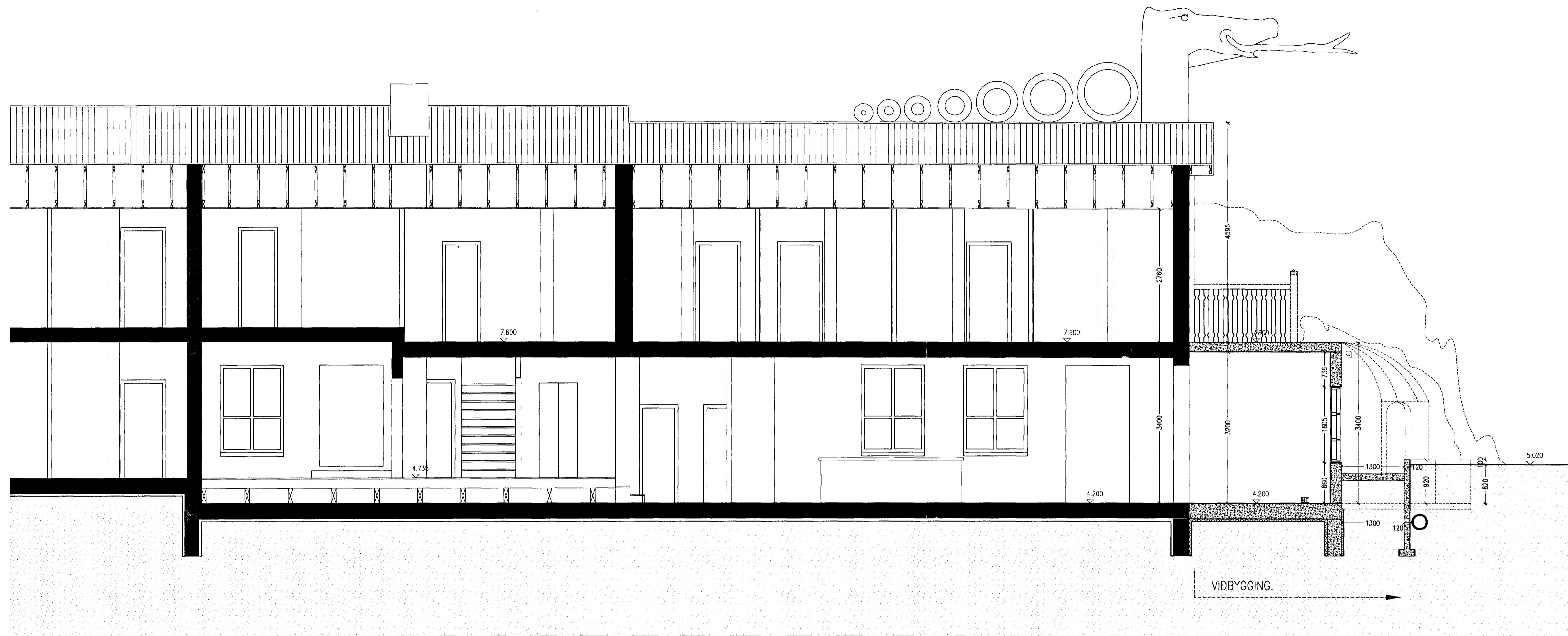
SNID D-D 1:50
