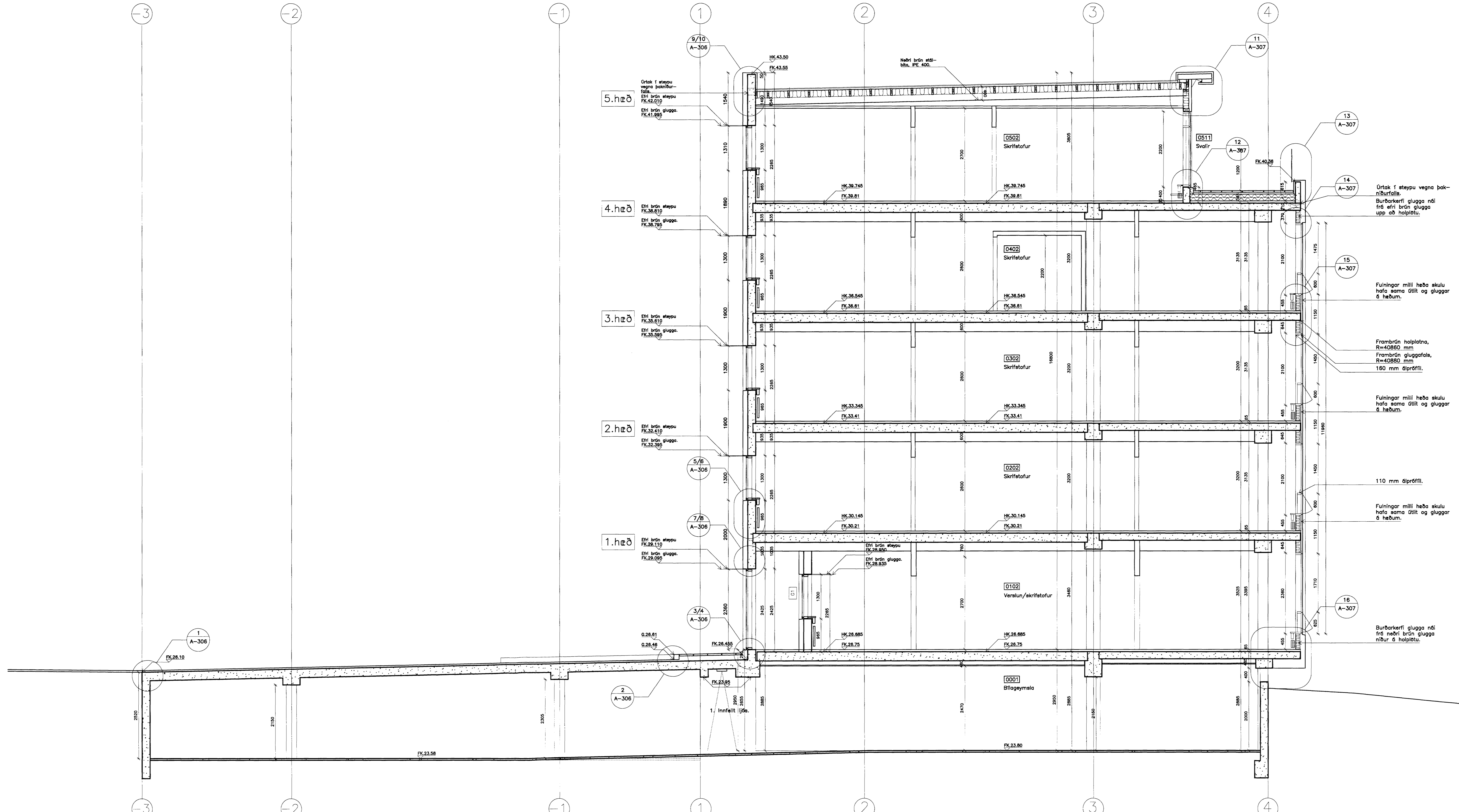
SNID A-A
