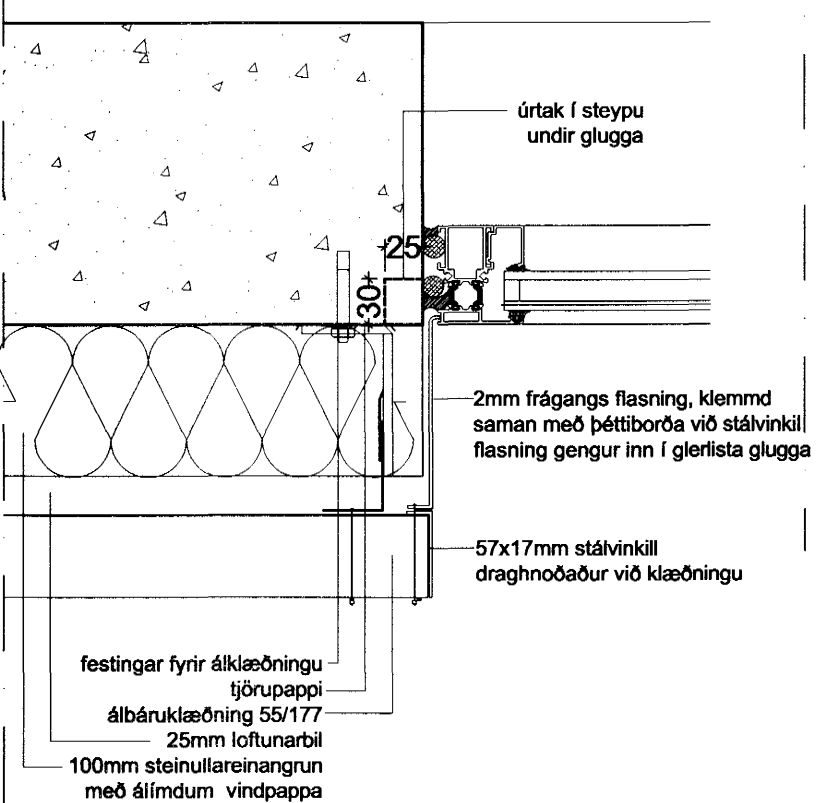
Frágangur við glugga/dyraop báruklæddra veggja Lárétt snið
