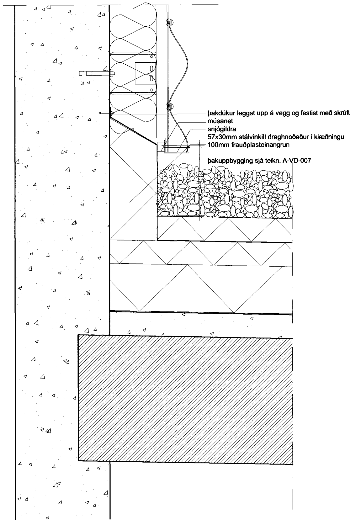
Frágangur við samskeyti flatra þaka og báruklæddra veggja Lóðrétt snið
