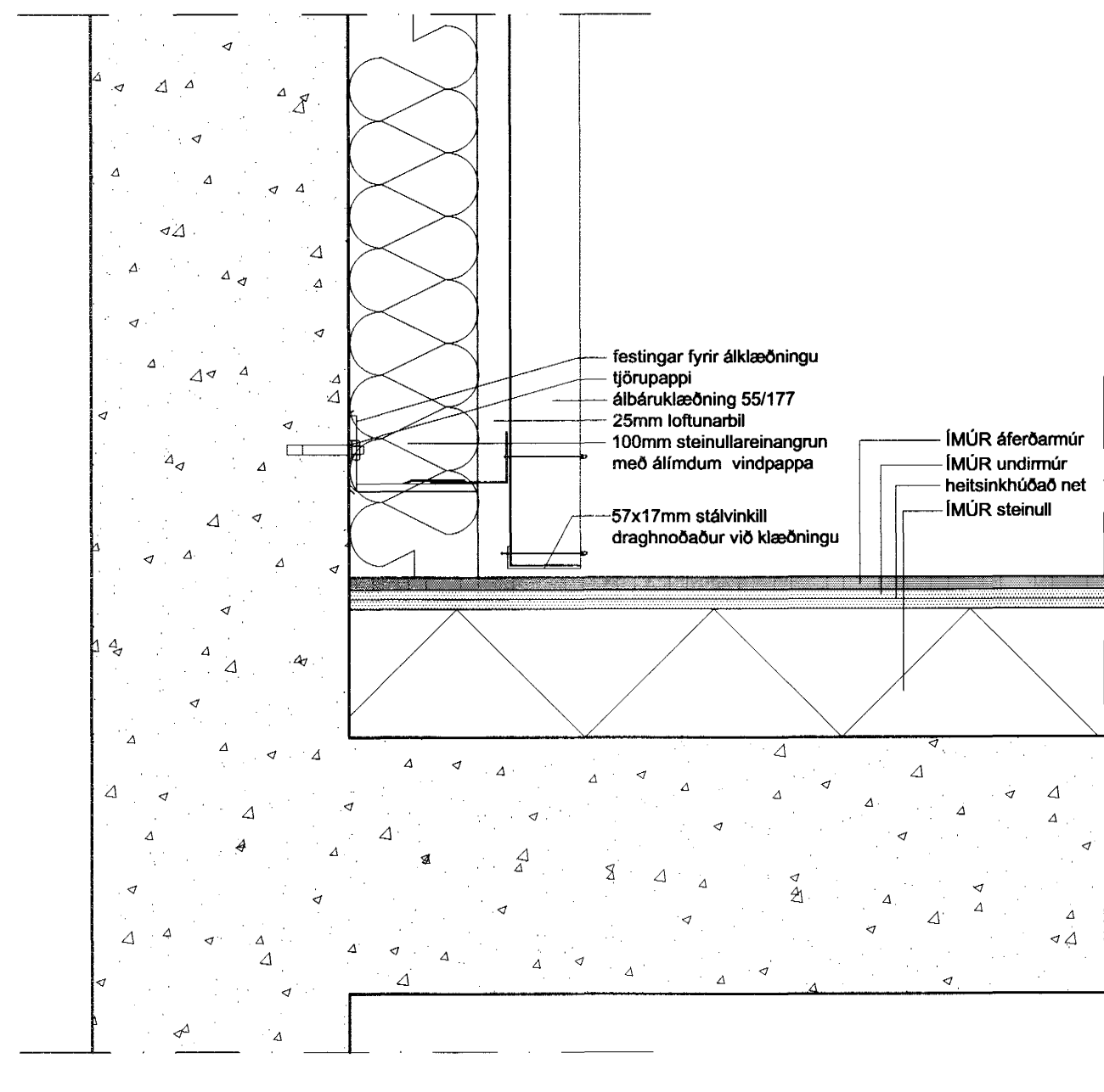
Frágangur við samskeyti ímúrklæðningar og báruklæðningar Lárétt snið
