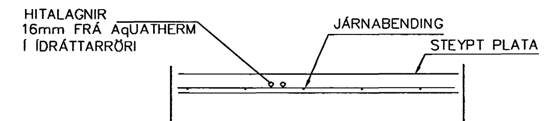
LAGNIR, SNIÐ, 1:20
