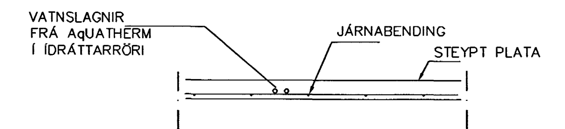
LAGNIR, SNIÐ, 1:20
