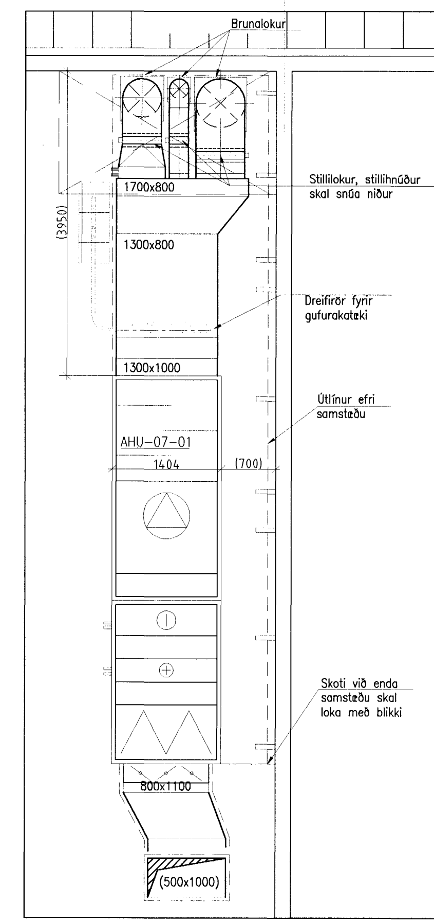
Grunnmynd - Samstæða AHU-07-01 Mkv. 1:50
