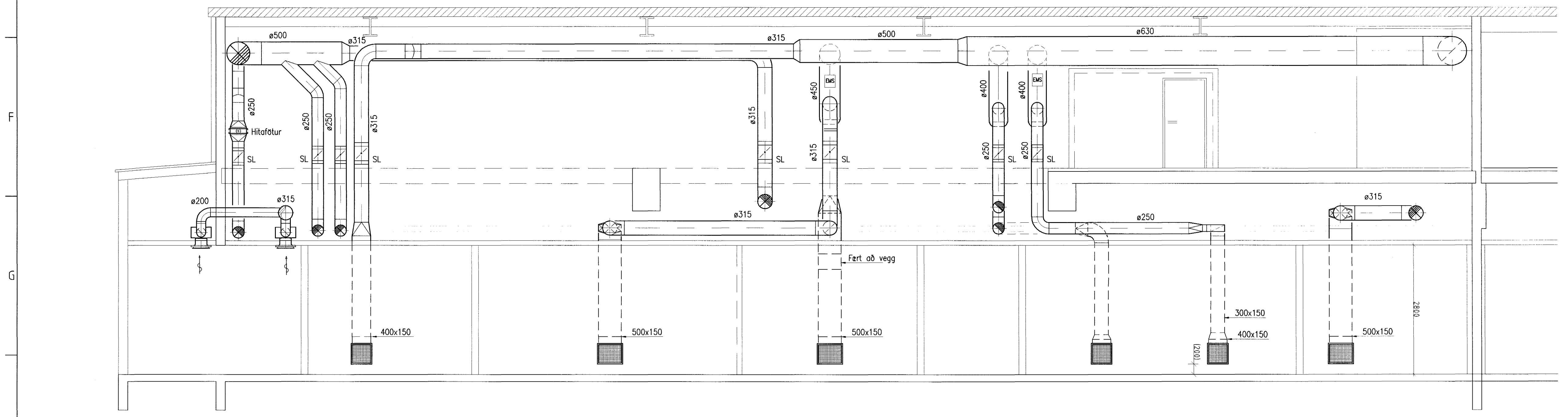
B Snið Mkv. 1: 50
