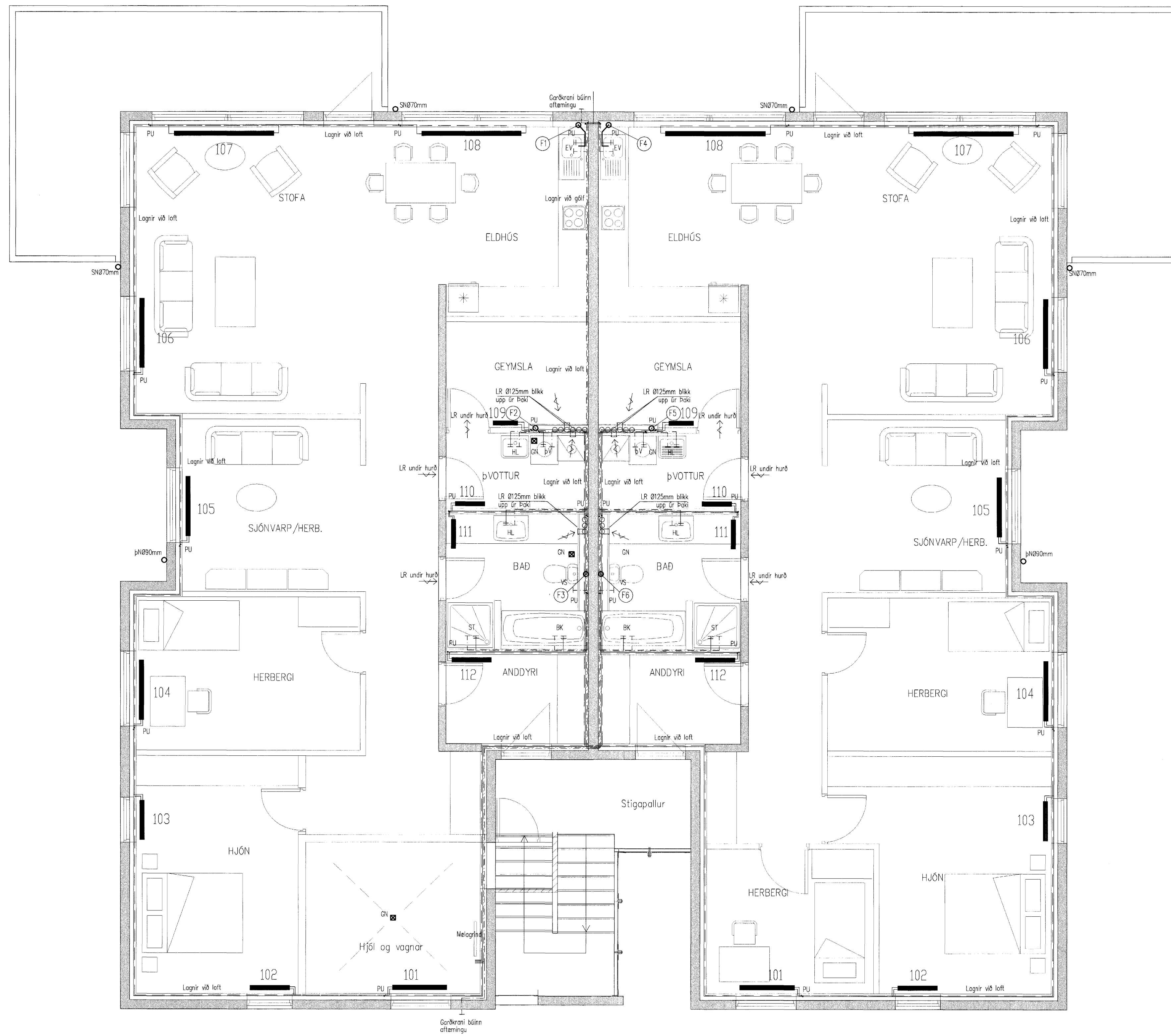
Grunnmynd 1 hæðar 1:50
