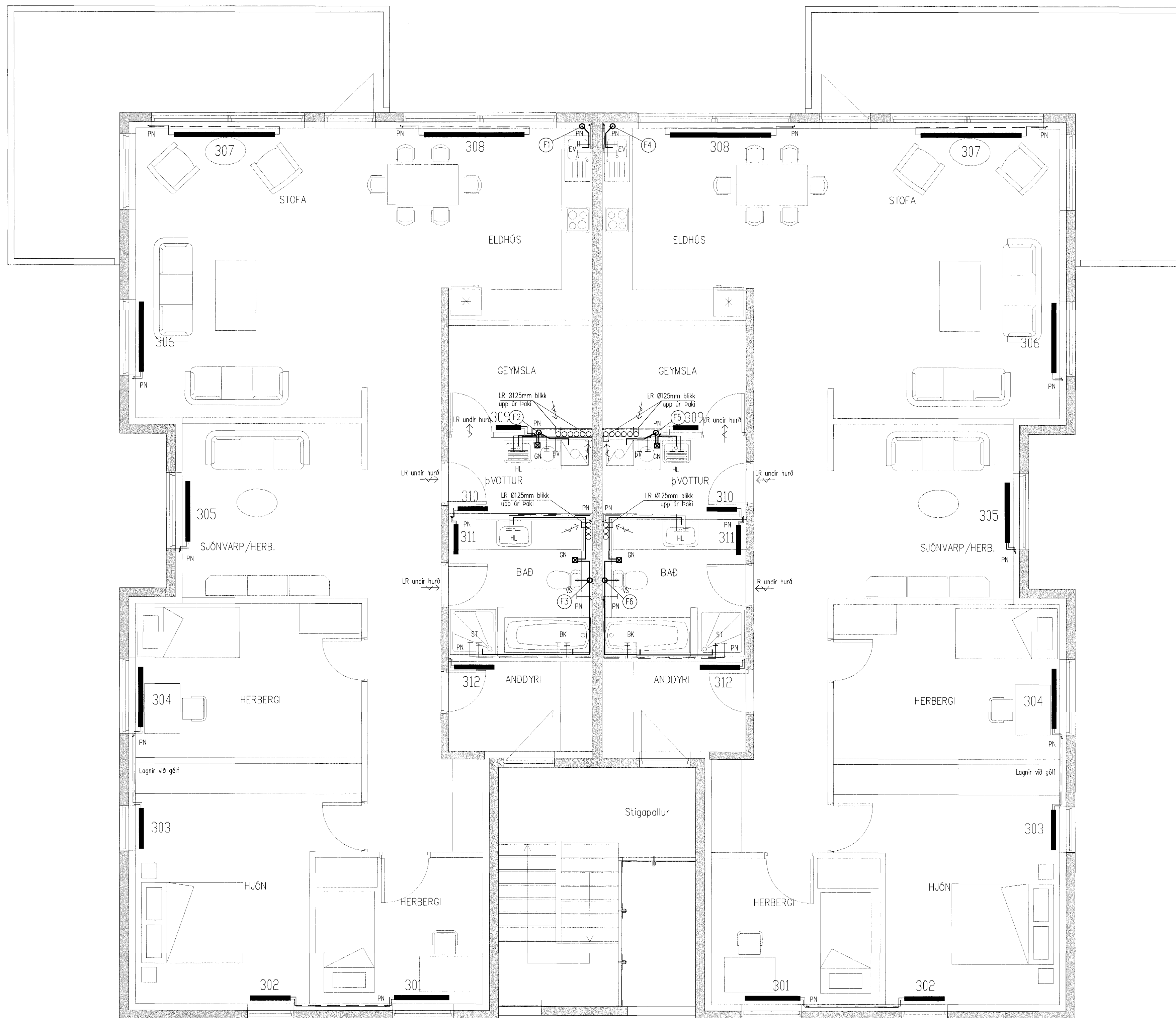
Grunnmynd 3 hæðar 1:50
