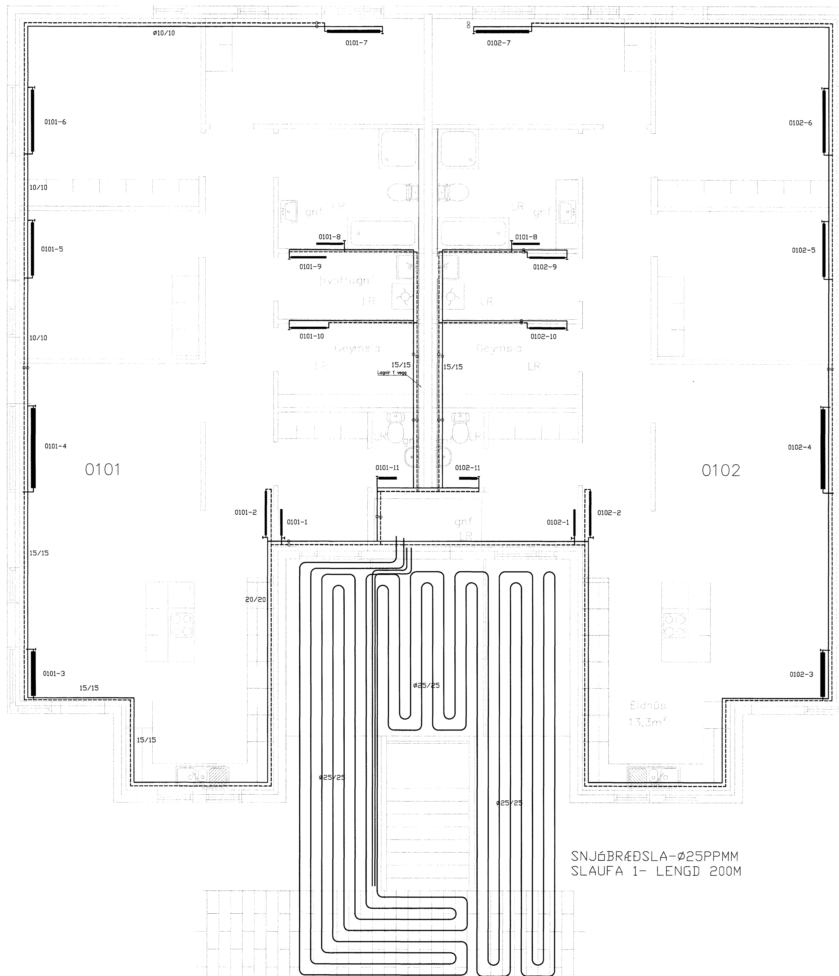
OFNALAGNIR OG SNJÓBRÆÐSLA, GRUNNMYND 1 HÆÐ 1:50
