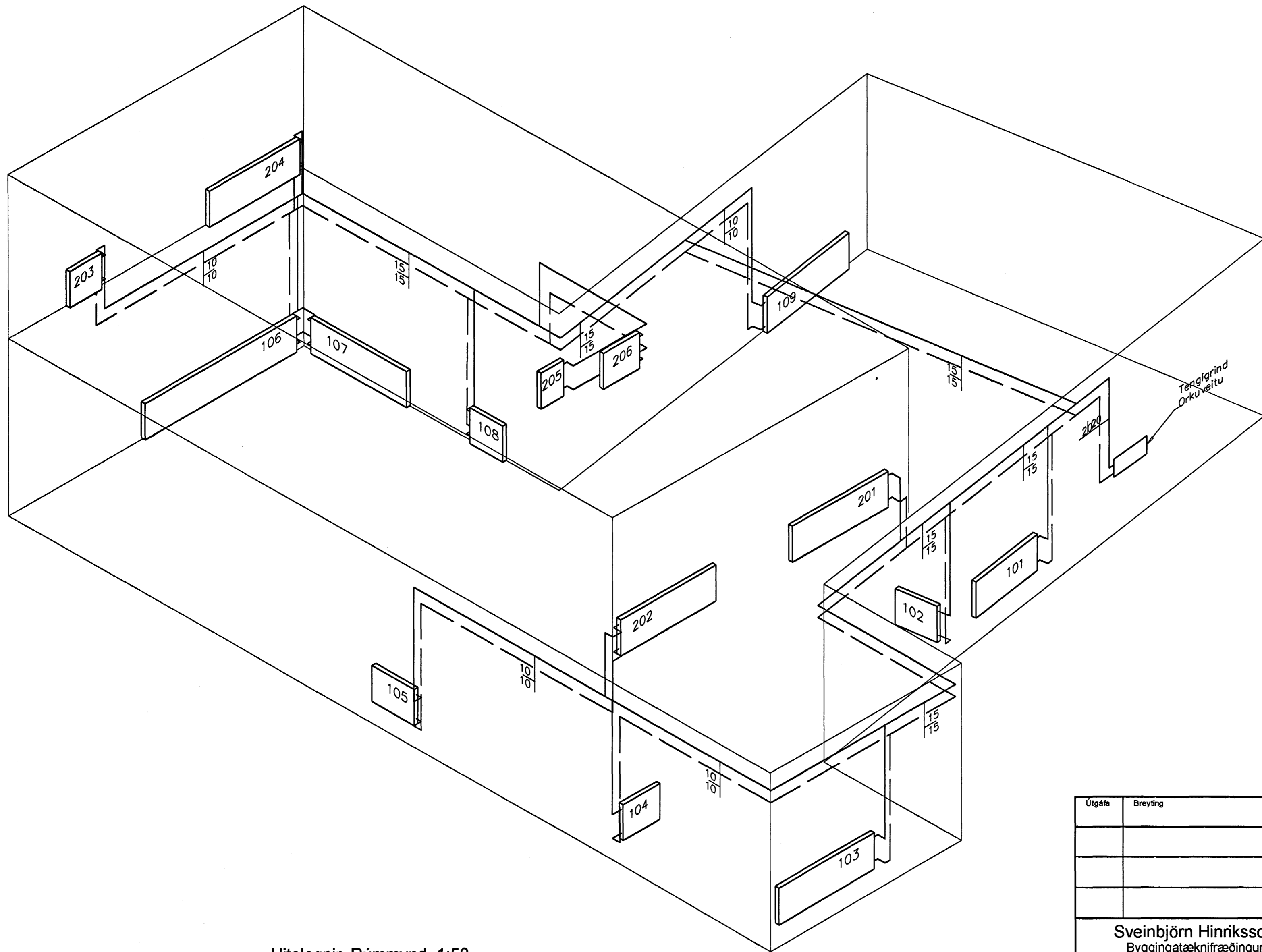
Hitalagnir, Rúmmynd, 1:50
