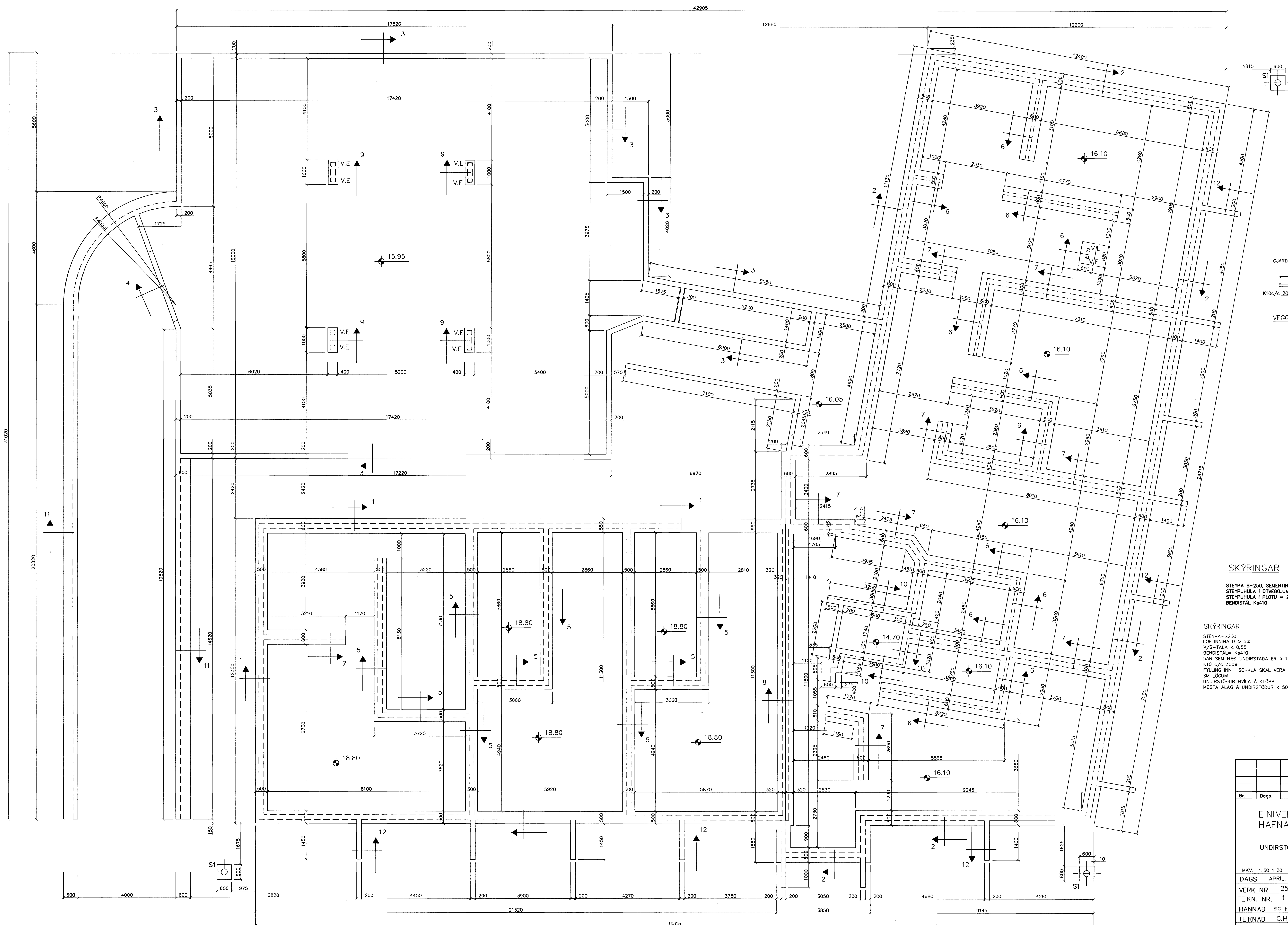
GRUNNMYND 1:50
