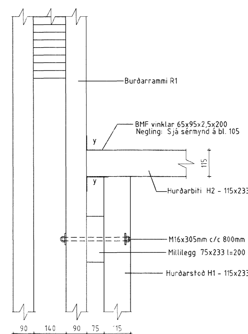
Sérmynd \gamma/24 Mkv.: 1:10
