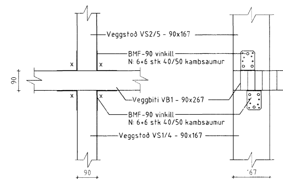
Sérmynd x/26 Mkv.: 1:10
