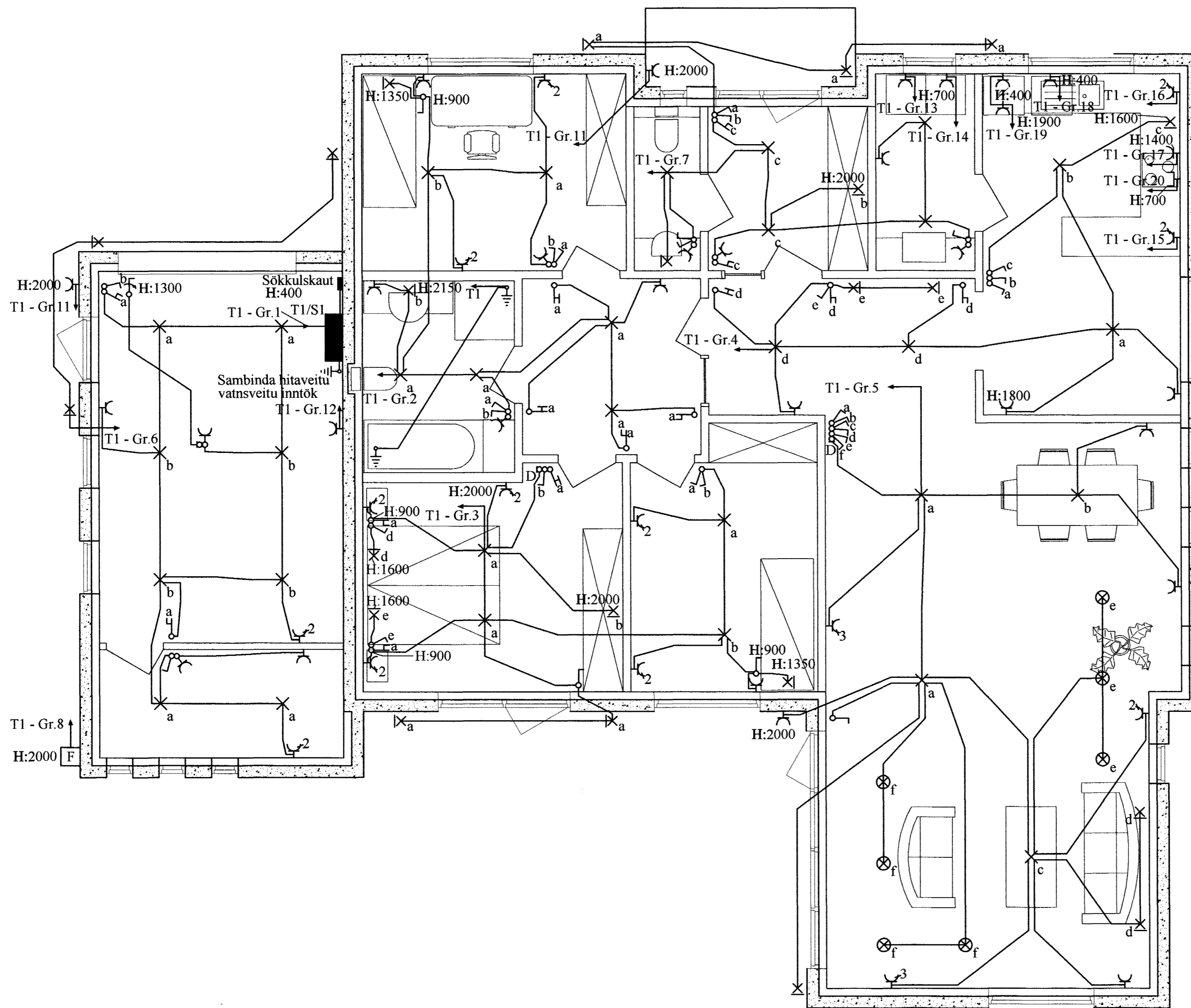
Grunnmynd - Raflögn
