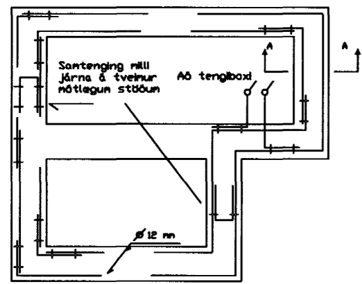
Grunnmynd Sökkulsveggja
