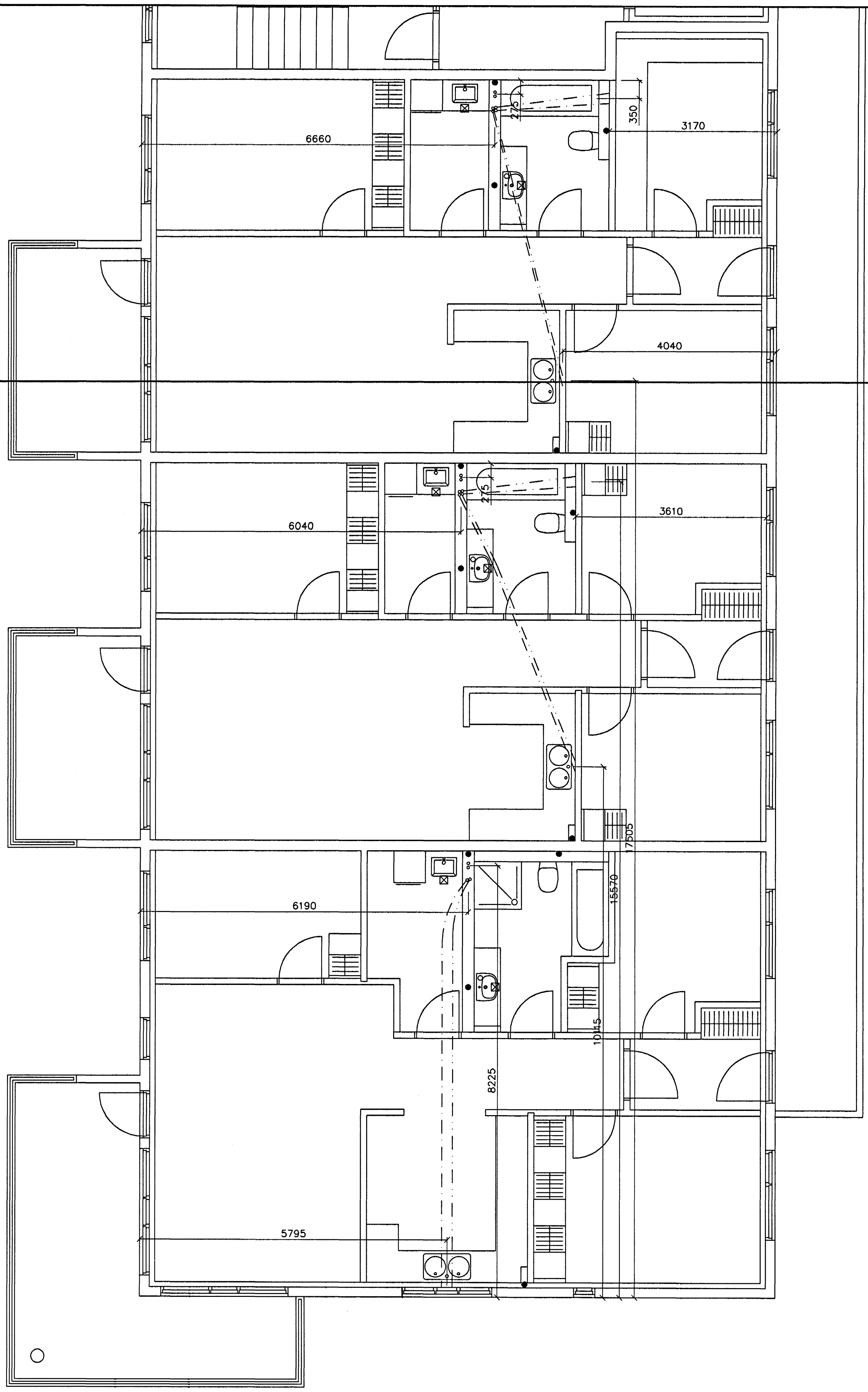
GRUNNMYND 3 HÆÐAR 1:50
