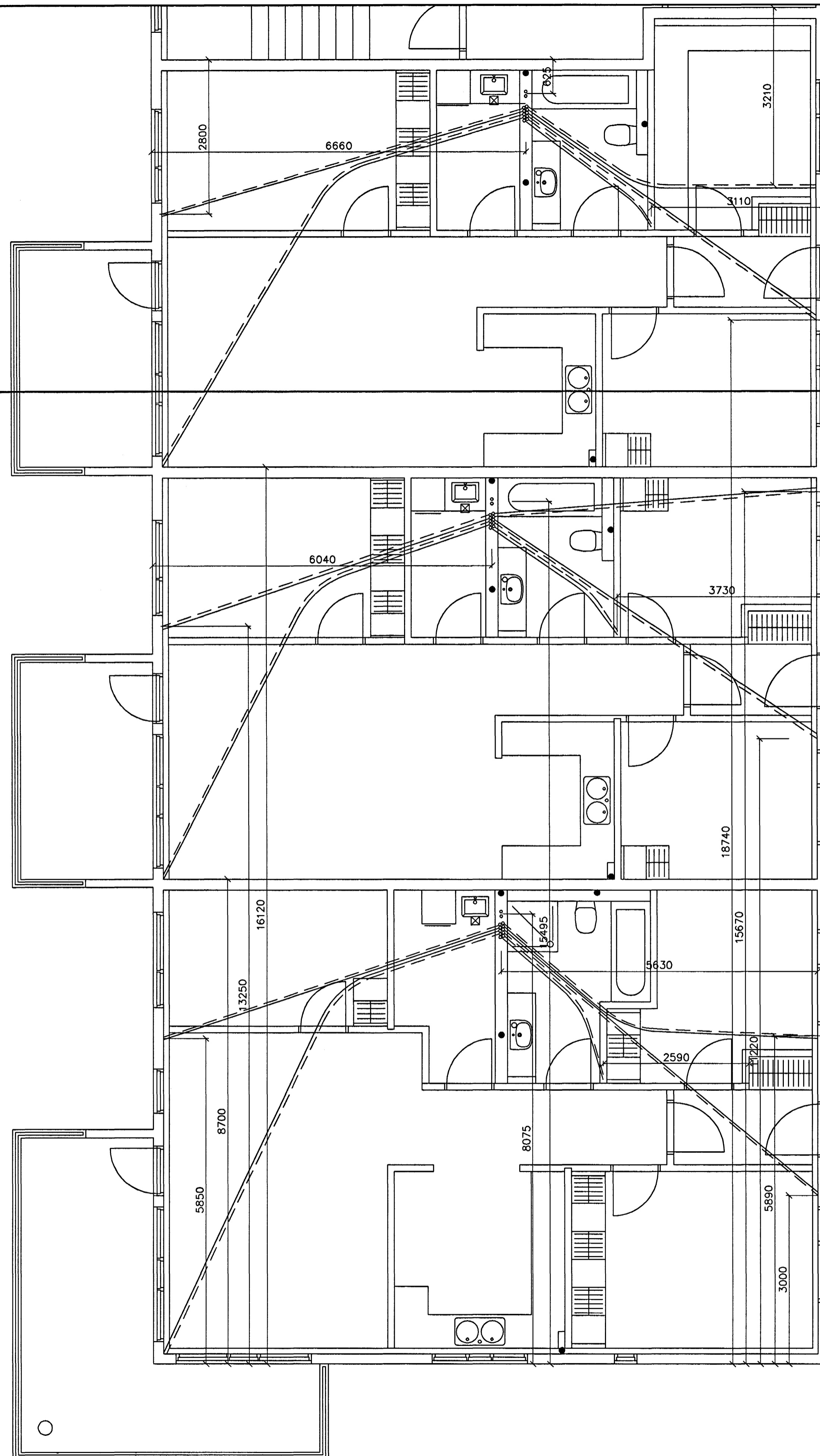
GRUNNMYND 3 HÆÐAR 1:50
