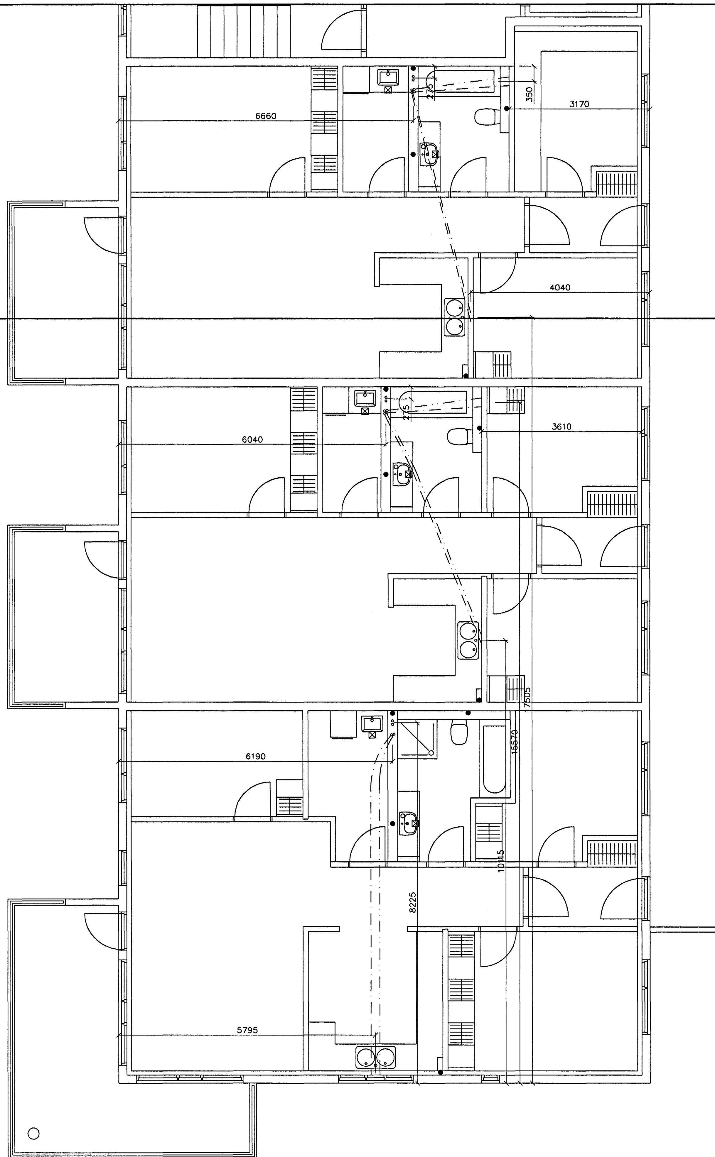
GRUNNMYND 4 HÆÐAR 1:50
