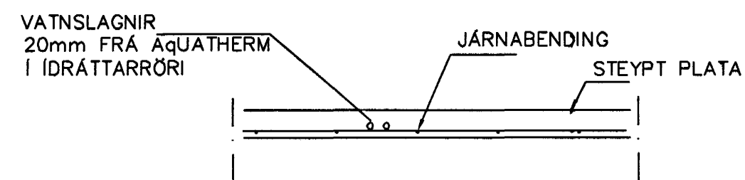
LAGNIR, SNIÐ, 1:20
